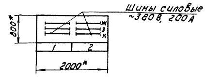
Вид А М 1:50
