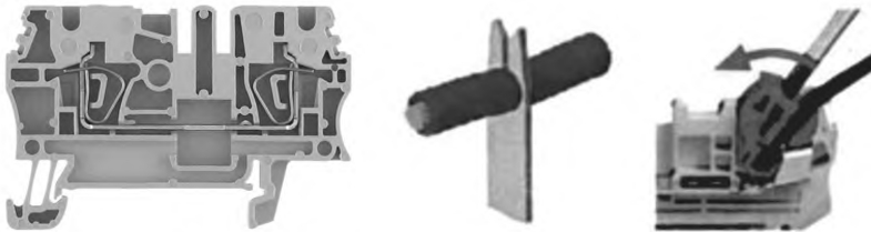
Рисунок 6.12 – Зажим в соответствии с технологией IDC
