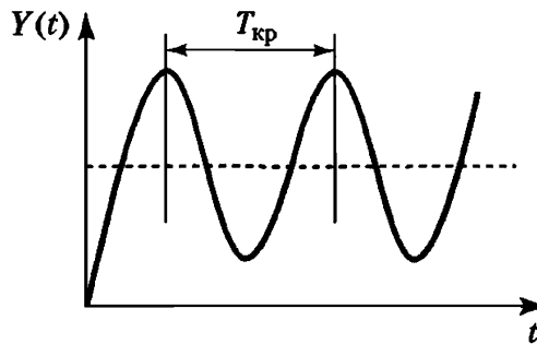
Рисунок 7.3 – Форма сигнала в методе незатухающих колебаний
