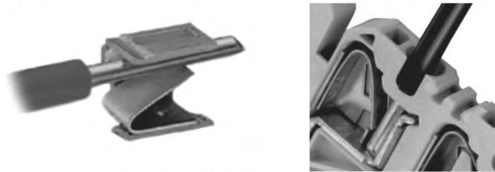
Рисунок 6.13 – Штекерный зажим
