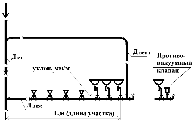
Рисунок 2 – Схема устройства длинной горизонтальной разводки
