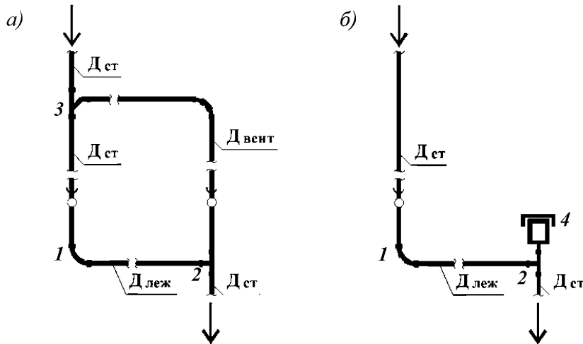
а) с устройством вентиляционного трубопровода (байпаса); б) с установкой автоматического противовакуумного клапана
