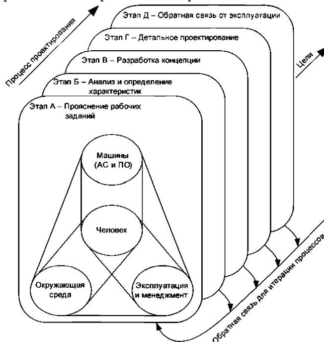
Рисунок II.1 – Итерационный подход к системному проектированию
