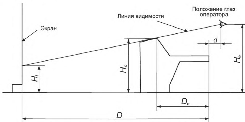
Рисунок П.6 – Элементы оборудования АРМ
