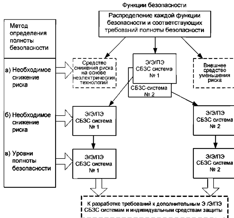
Рисунок 6 – Распределение требований безопасности по Э/Э/ПЭ СБЗС системам, средствам снижения риска не основе неэлектрических технологий и внешним средствам уменьшения риска
