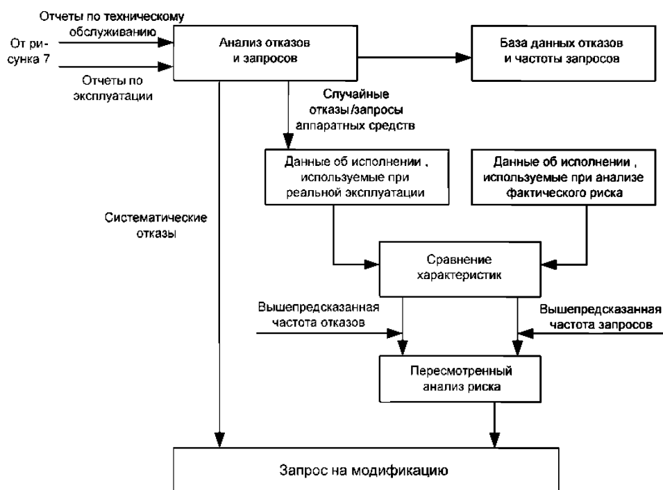
Рисунок 8 – Пример модели управления эксплуатацией, ТО и ТР
