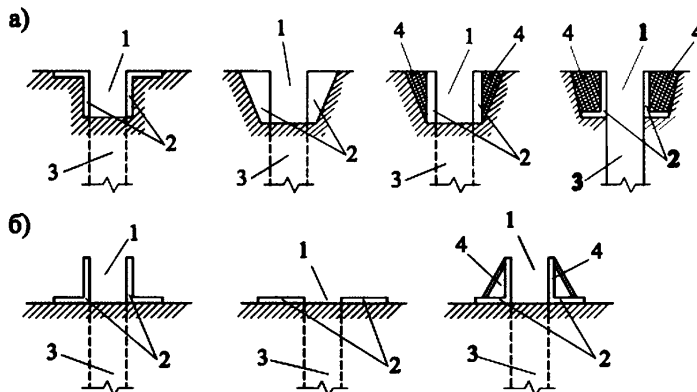
а) заглубленная формашта; б) наземная формашта
