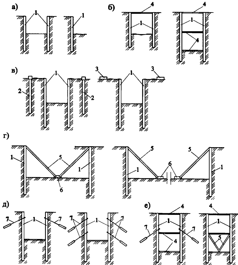
а) консольный; б) распорный; в) удерживающий; г) подпорный; д) анкерный; е) комбинированный
