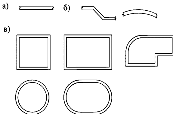
Рисунок 3 – Типовые схемы конфигурации СГ в плане
