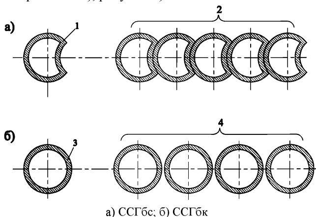
Рисунок 5 – Типовая форма поперечного сечения обсадной трубы для устройства ССГ
