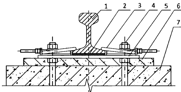
1-направляющая; 2-упругая прокладка; 3-промежуточное крепление УПК-1; 4-анкерный болт; 5-опорная плита; 6-подливка безусадочного раствора; 7-монолитное железобетонное основание
