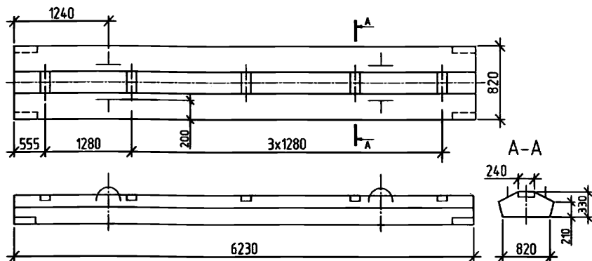
Рисунок ПВ.3- Железобетонная балка БРП – 62.8.3
