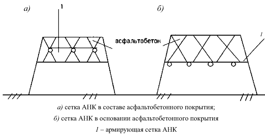
Рисунок Д.3 – Варианты армирования асфальтобетонного покрытия
