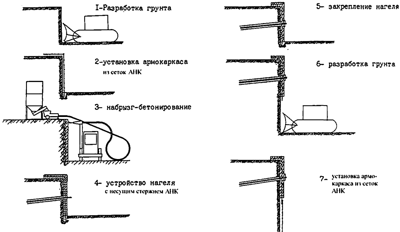
Рисунок 8.13 – Технология устройства нагельного крепления с набрызг-бетонным экраном и буронагельным нагелем с несущим стержнем АНК
