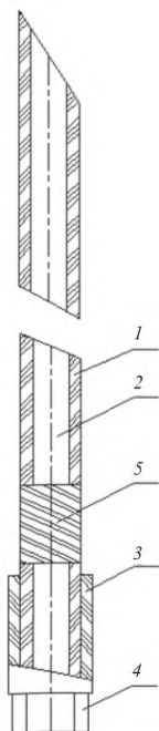
1 – стержень АНК-С трубчатого сечения; 2 – внутренний канал; 3 – втулка; 4 – торец нижний граненый; 5 – опорная пластина
