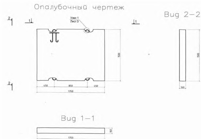
Рисунок Д.1 – Опалубочный чертеж дорожной плиты
