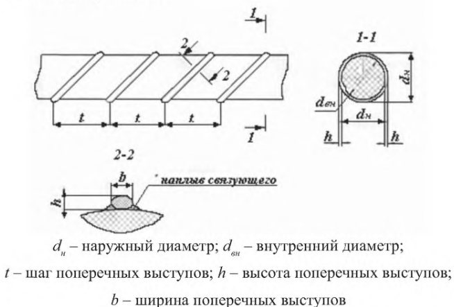
Рисунок 4.1 – Типовое сечение АНК с рельефной боковой поверхностью периодического профиля
