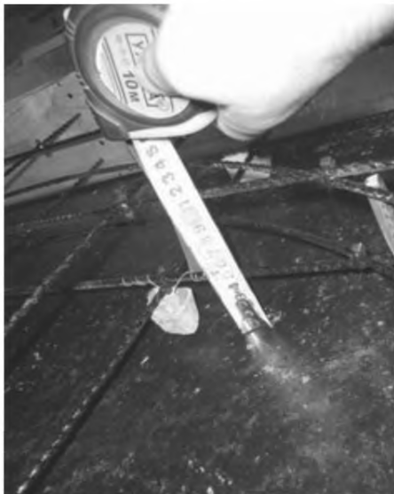
Рисунок 6.3 – Фрагменты арматурных каркасов из базальтопластиковых стержней, уложенных в опалубочную форму дорожной плиты с контролем их геометрических параметров
