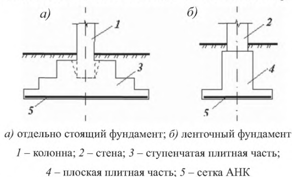
Рисунок 8.2 – Схема армирования фундаментной плиты
