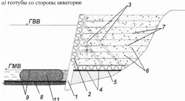
Рисунок 8.23 – Сооружение буны с использованием композитной арматуры 1)
