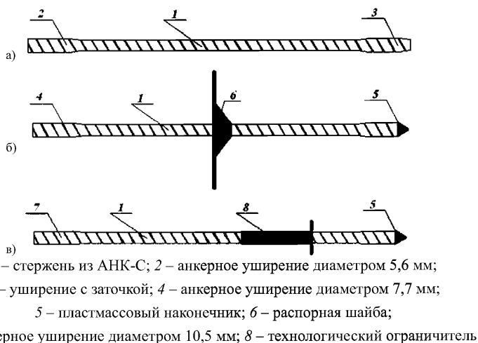
Рисунок 7.3 – Конструкции гибких связей из АНК-С
