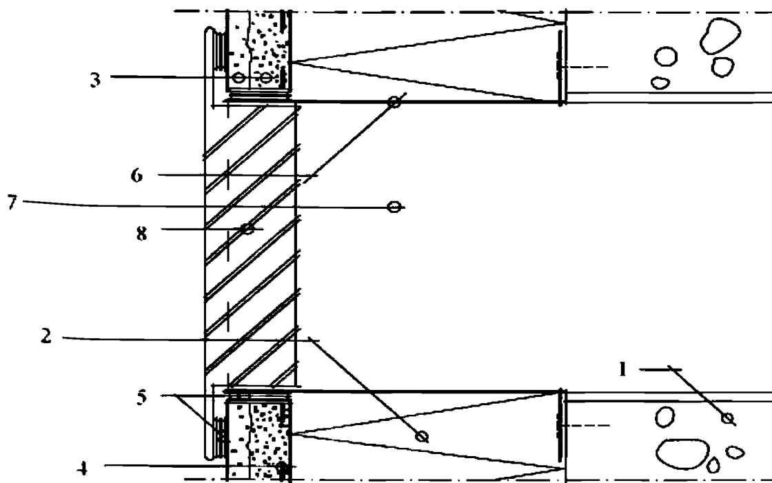
1 – наружная стена; 2 – теплоизоляционный слой; 3 – штукатурный слой; 4 – армирующая сетка; 5 – эластичная шовная мастика вокруг решетки; 6 – наставка воздуховода; 7 – воздуховод, 8 – вентиляционная решетка
