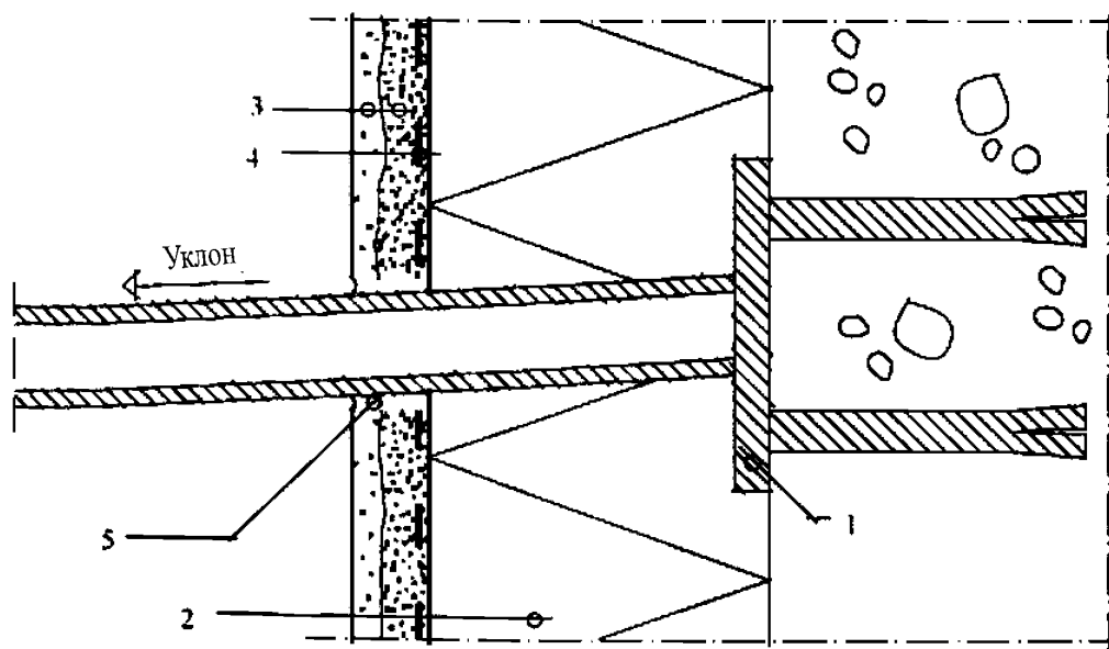
1 – крепление лестниц к стене (по проекту конструктора); 2 – теплоизоляционный слой; 3 – штукатурный слой; 4 – армирующая сетка; 5 – эластичная шовная мастика вокруг трубы
