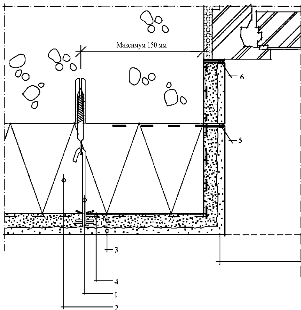
1 – шарнирный анкер; 2 – теплоизоляционный слой; 3 – штукатурный слой; 4 – армирующая сетка; 5 – деформационный шов (ширина 4 – 6 мм, материал – эластичная шовная мастика); 6 – эластичная шовная мастика
