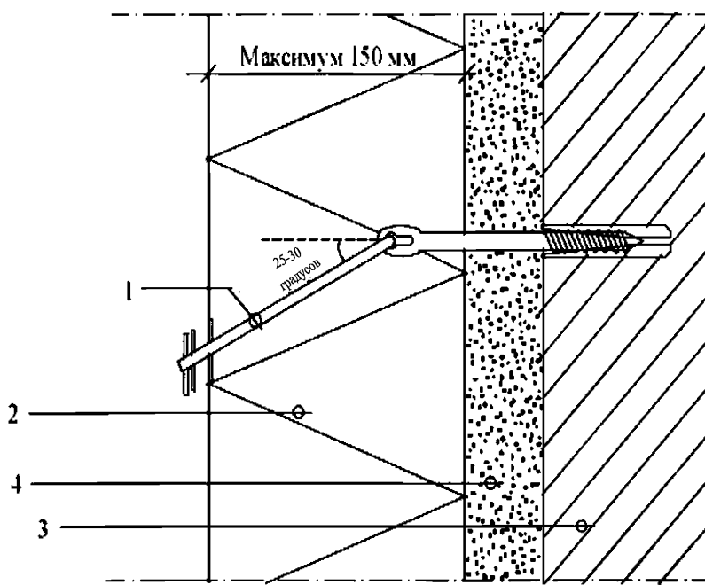
1 – шарнирный анкер; 2 – теплоизоляционный слой; 3 – основание
