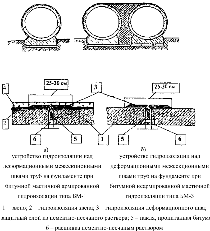
Рисунок К.3 – Устройство гидроизоляции водопропускных труб
