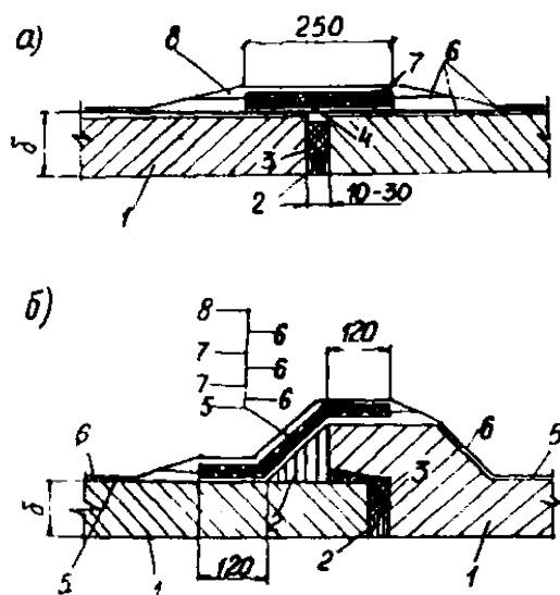
а) фальцевый стык звеньев труб; б) раструбный стык звеньев труб
