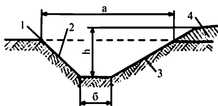
б) Кювет трапециевидального сечения
