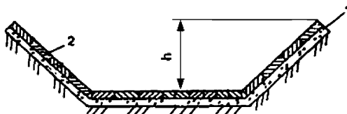
Рисунок 7 – Быстоток, укрепленный цементобетонными плитами
