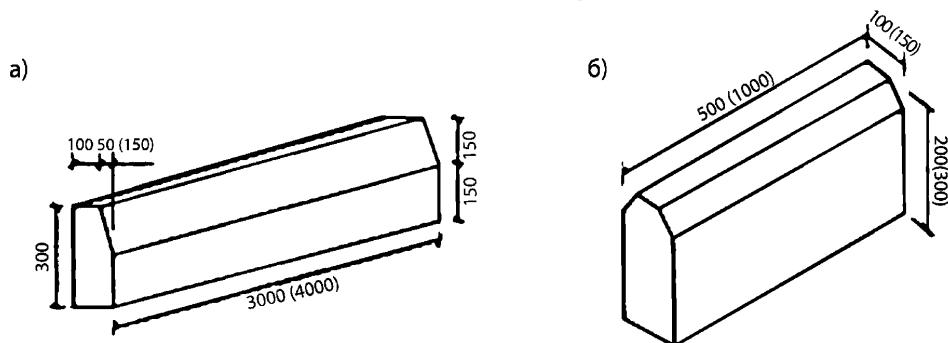
Рисунок В.1 – Геометрические параметры типовых бордюрных блоков
