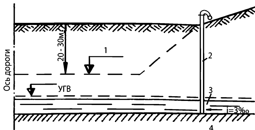
Рисунок Д.1 – Установка иглофильтров
