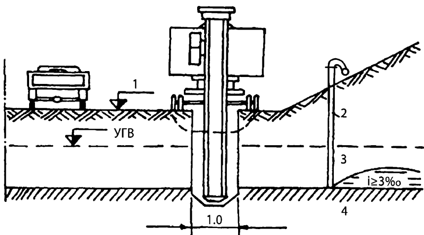
Рисунок Д.1 – Установка иглофильтров
