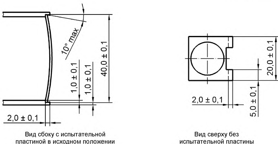
Рисунок 5 – Зажимы
