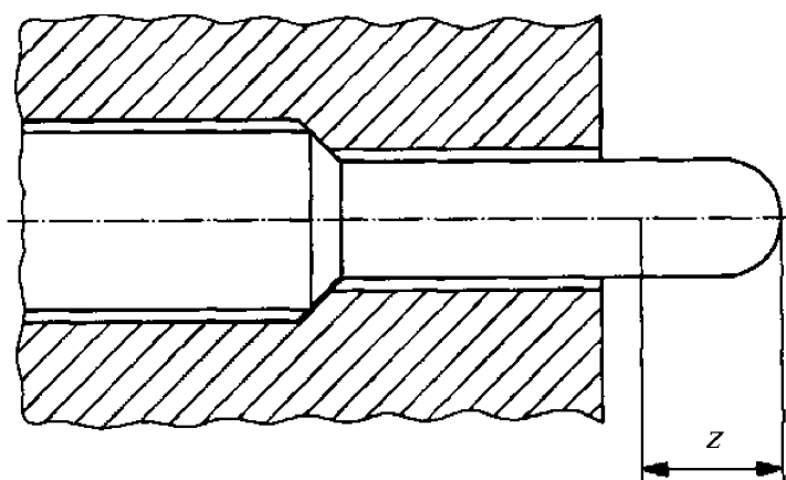
Рисунок 1 – Испытательная установка
