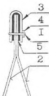
Сшивка через наклеенную ленту; лента под швом
