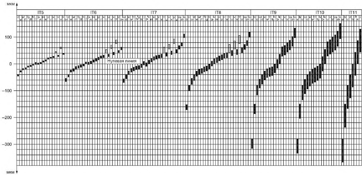
Рисунок А.4 — Графическое представление классов допусков валов в зависимости от диаметров
