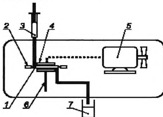
1 – камера для образца; 2 – оптическое детектирование; 3 – шприц вместимостью 10 см 3 ; 4 – испытательная ячейка; 5 – миниатюрный компрессор; 6 – устройство измерения температуры; 7 – контейнер для отходов Рисунок А1.2 – Схема аппарата
