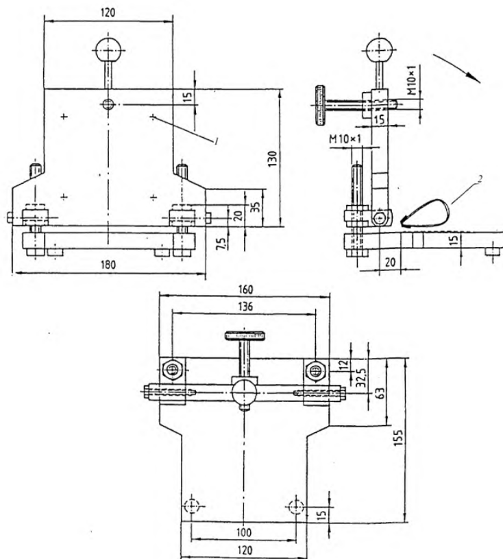
Рисунок 1 – Фальцовочный аппарат (пример)
