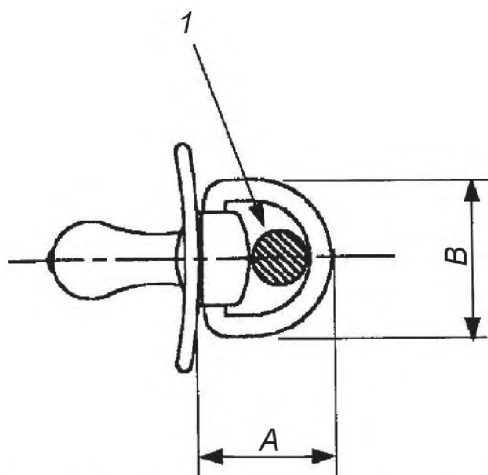
Рисунок 13 – Размеры кольца
