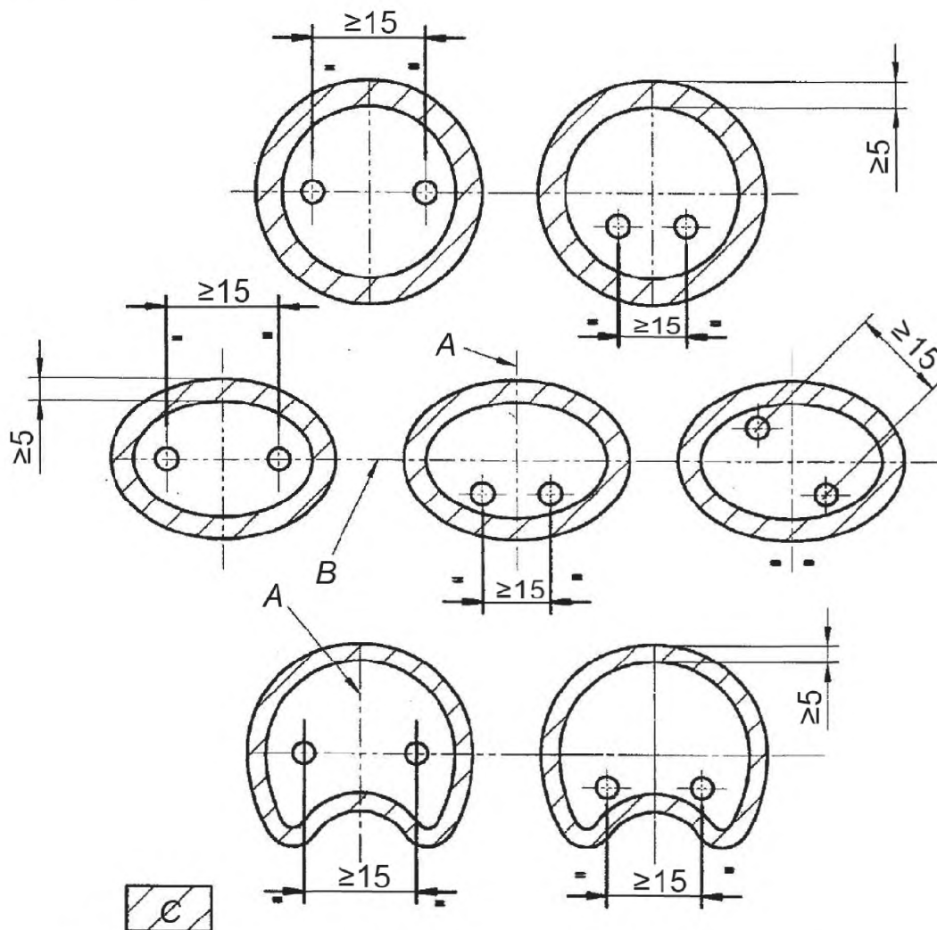
А – малая ось; В – основная ось; С – заштрихованная область – допускаемые отверстия Рисунок 10 – Примеры размещения допускаемых отверстий (5.2.3.1)
