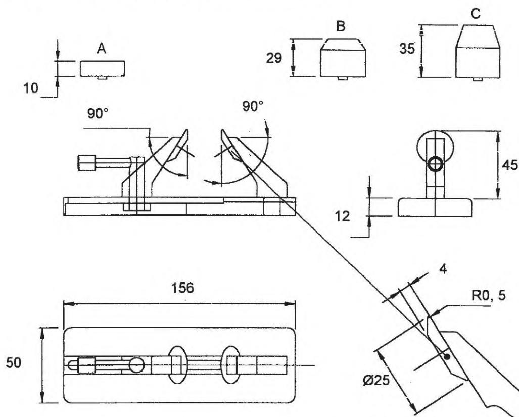
А – эталонная плитка А; В – эталонная плитка В; С – эталонная плитка С Рисунок 5 – Пример приспособления для определения длины баллончика
