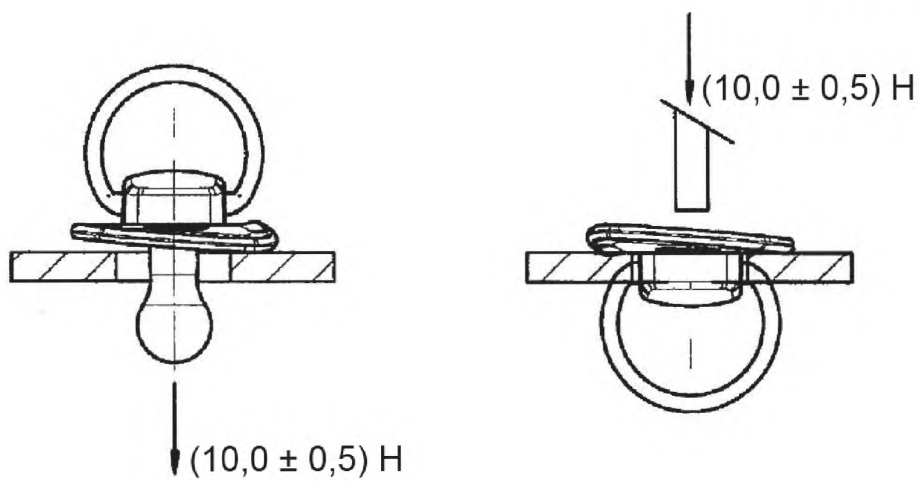
Рисунок 11 – Испытание защитного диска (5.2.3.2)
