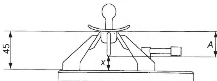
A – размер A; x – расстояние между нижней поверхностью кольца и верхней поверхностью эталонной плитки
