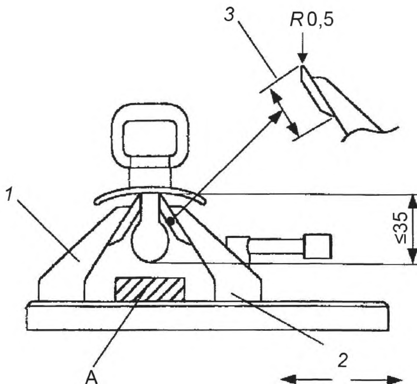
A – эталонная плитка A; 1 – неподвижный зажим; 2 – подвижный зажим; 3 – диск диаметром 25 мм
