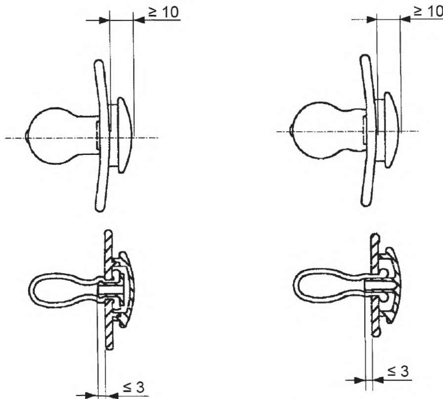
Рисунок 15 – Измерение расположения головки, пробки, крышки
