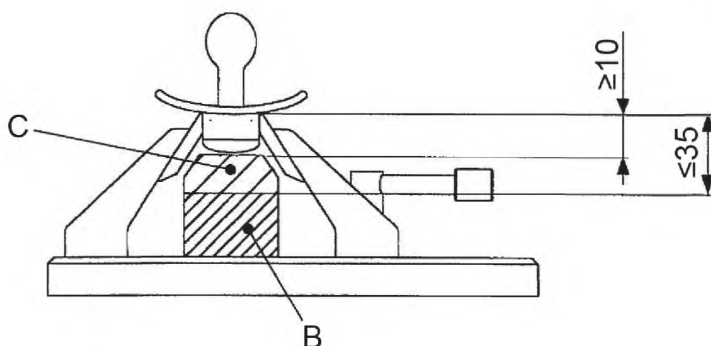
В – эталонная плитка В; С – эталонная плитка С Рисунок 8 – Эталонная плитка для определения длины головки
