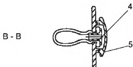
1 – баллончик; 2 – защитный диск; 4 – пробка; 5 – крышка; 7 – поверхность защитного диска, обращенная ко рту ребенка Рисунок 3 – Соска с пробкой и крышкой
