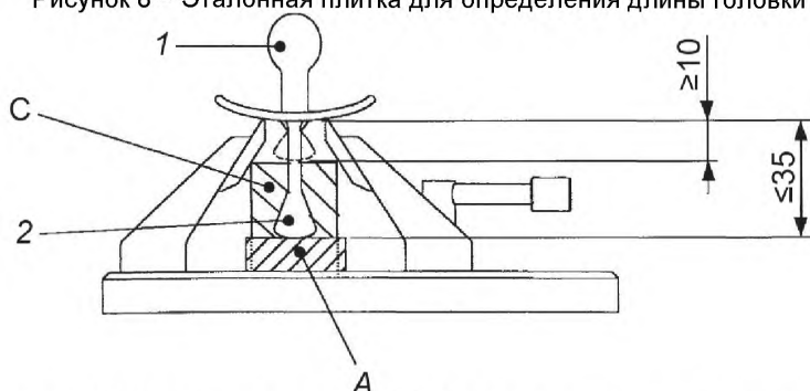
А – эталонная плитка А; С – эталонная плитка С; 1 – баллончик соски; 2 – эластичное кольцо или головка
