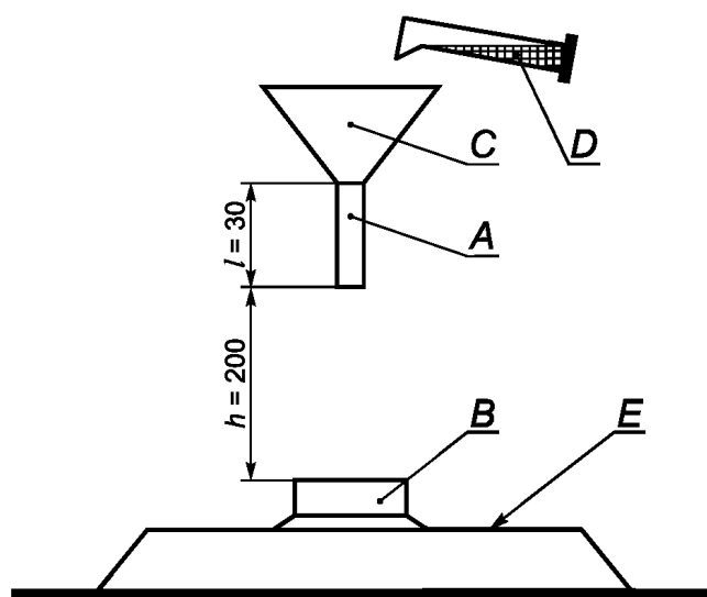
Рисунок 102 — Защитные устройства для машин для нарезки ломтиков
