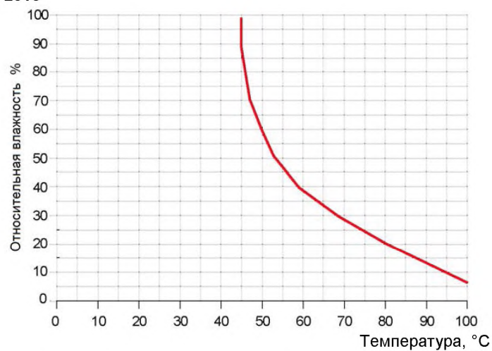
Рисунок 101 – Характеристика температуры/относительной влажности при нормальной работе
