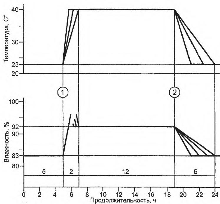
Рисунок 102 – График температуры и влажности
