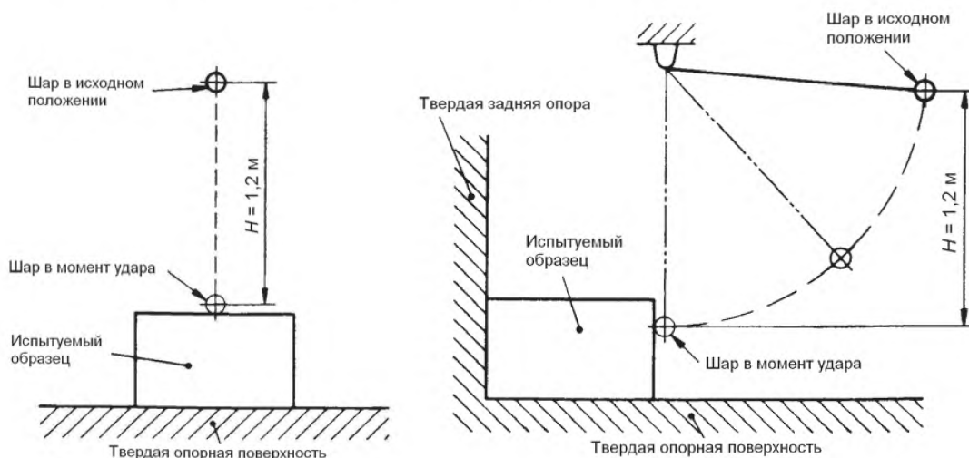
Рисунок 101 – Испытания на удар с помощью стального шара
