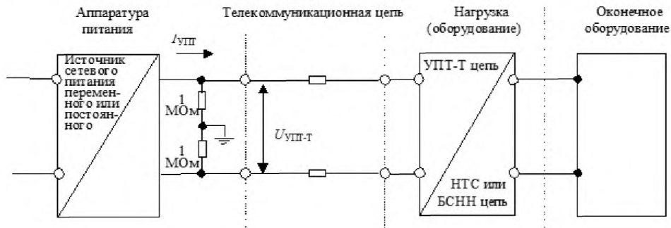
Рисунок А.1 – Пример УПТ-Т системы удаленного электропитания
