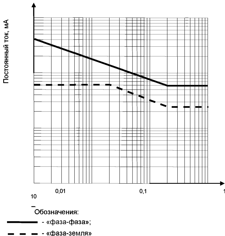
Рисунок 1 – Максимальный ток после единичной неисправности
