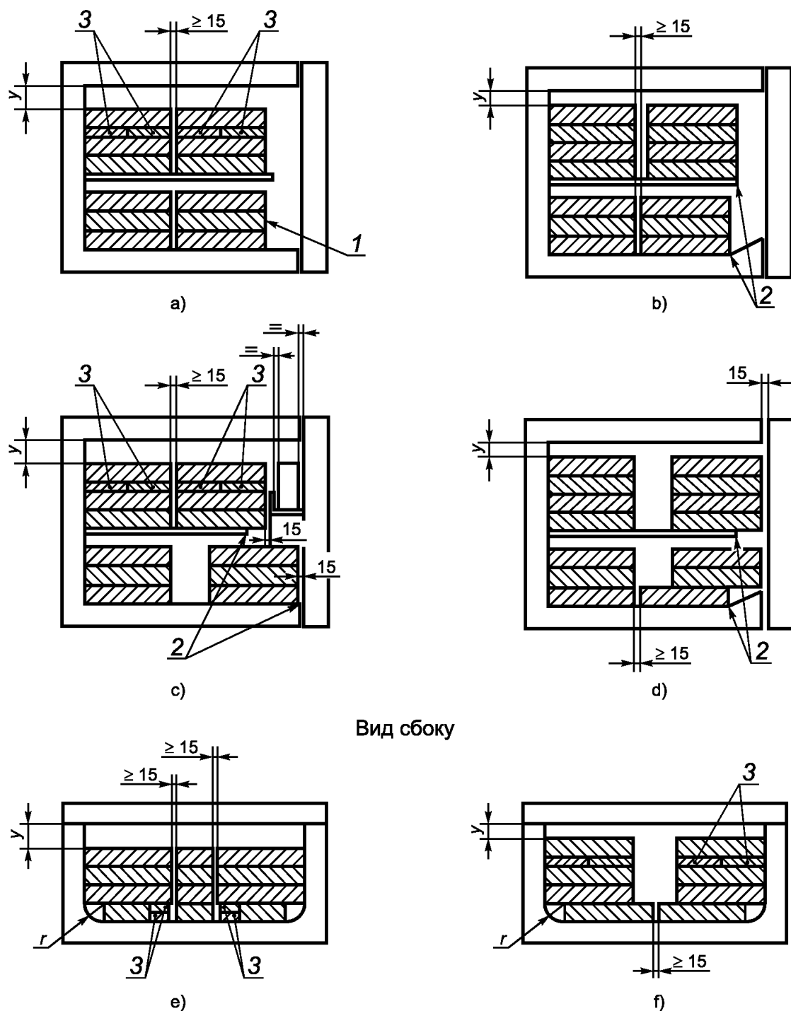
Вид спереди (емкости со скругленными углами)
