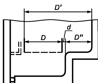
д) Определение глубины полки, состоящей из элементов, установленных друг против друга
