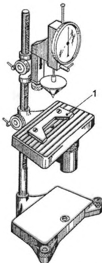
1 – центрирующее устройство
