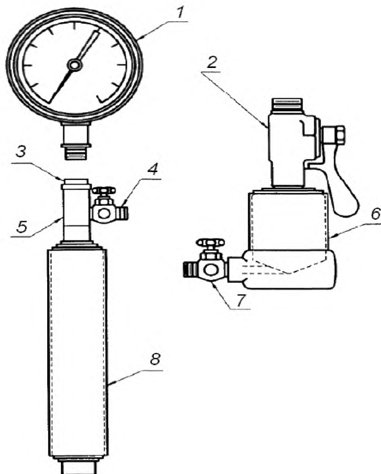
1 – манометр; 2 – проходной кран; 3 – соединение манометра; 4 – вентиль для продувки; 5 – соединение вентиля для продувки; 6 – нижняя камера; 7 – впускной вентиль; 8 – верхняя камера
