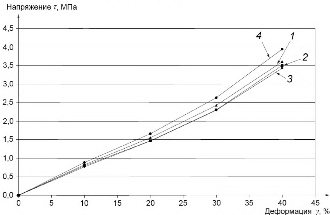
Рисунок А.1 – Статические упругопрочностные свойства при сжатии образцов на пластинках со смазкой (напряжения приведены без поправок)
