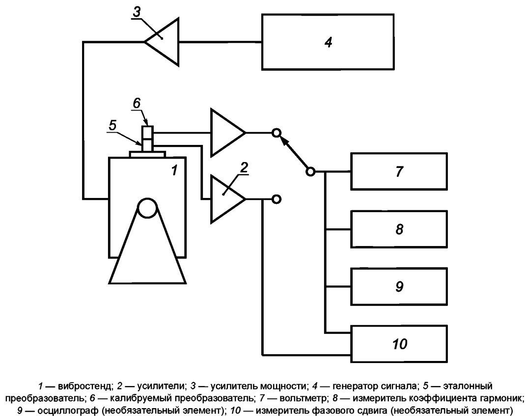
Рисунок 1 — Блок-схема испытательной установки для вибрационной калибровки сравнением с эталонным преобразователем
