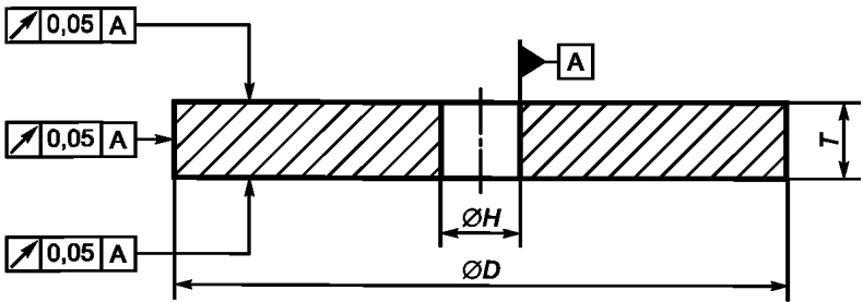
D — внешний диаметр; H — диаметр отверстия; T — толщина
