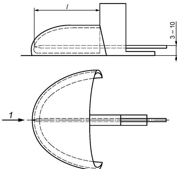
Рисунок 3 — Измерение внутренней длины подноски
