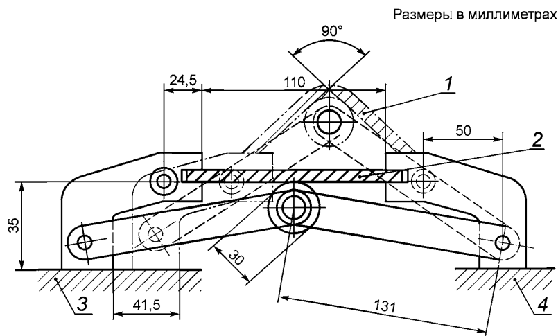
Рисунок 33 — Испытательное устройство для испытания подошвы на изгиб
