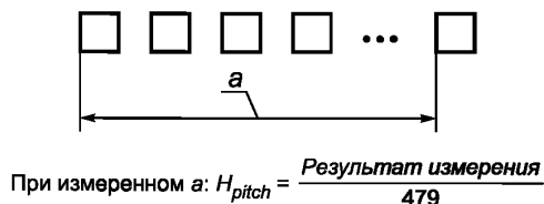
Рисунок 62 — Измерение шага пикселя по изображению на дисплее
