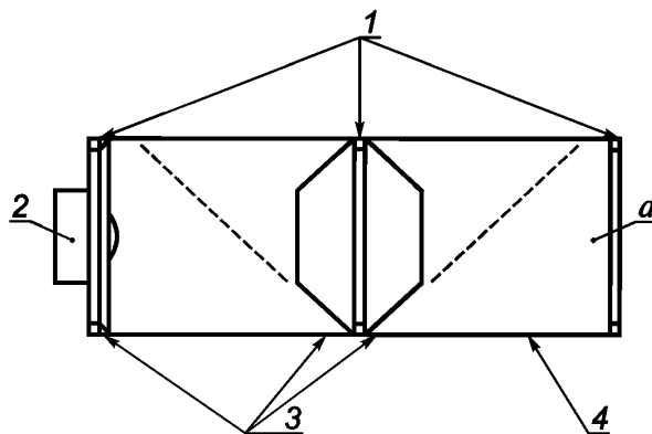
1 — кольца; 2 — прибор измерения освещенности; 3 — черные глянцевые конусы; 4 — черная глянцевая трубка; a — со стороны проектора
