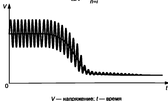
Рисунок 53 — Кривая переходной характеристики (SRF) с периодической пульсацией
