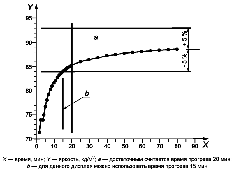
Рисунок 56 — Время прогрева
