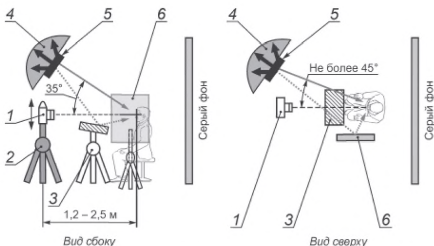
1 — камера; 2 — штатив; 3 — отражающая панель; 4 — ламповый отрагатель; 5 — источник освещения; 6 — боковая отражающая панель
