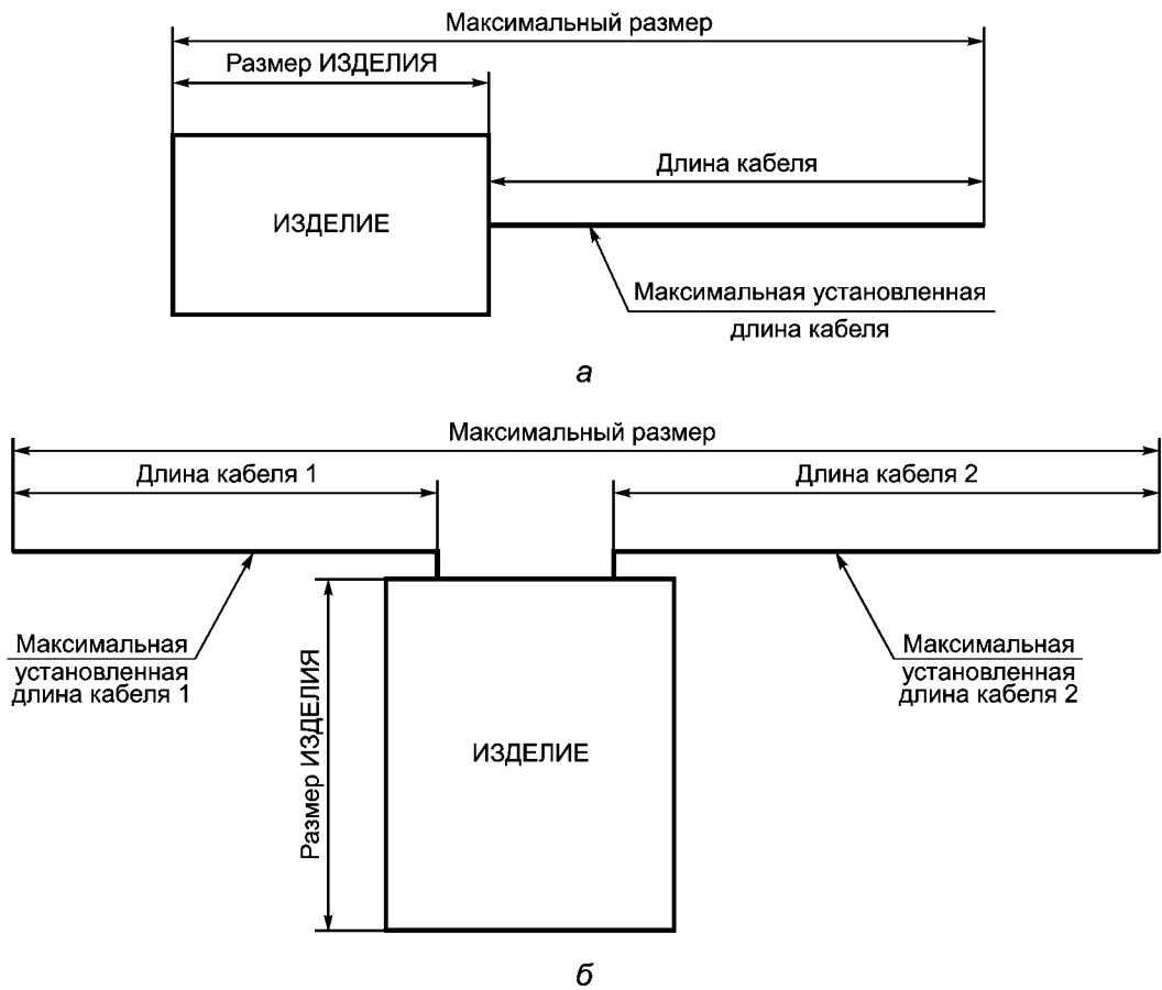
Рисунок А.2 — Примеры определения максимальных размеров МЕ ИЗДЕЛИЙ [см. 6.2.6.1 е) и f)]: а — с одним кабелем; б — с двумя кабелями
