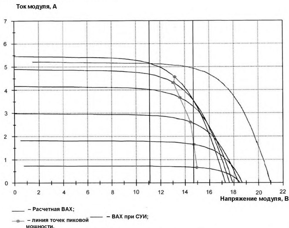
Рисунок С.2 – Набор ВАХ, соответствующий дневному профилю энергетической освещенности
