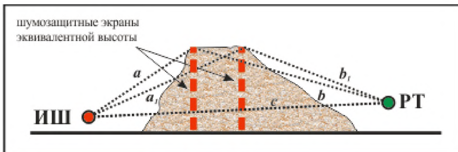
Рисунок 11.18 - Схемы расчета акустической эффективности шумозащитного вала
