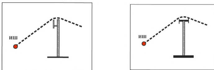
Рисунок 11.13- Схемы кранов с уширенной верхней частью, повышающие акустическую эффективность
