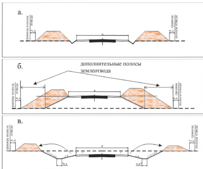
Рисунок 11.50 - Шумозащитные валы в нулевых отметках (а), на участке насыпи (б) и на участке выемки (в)
