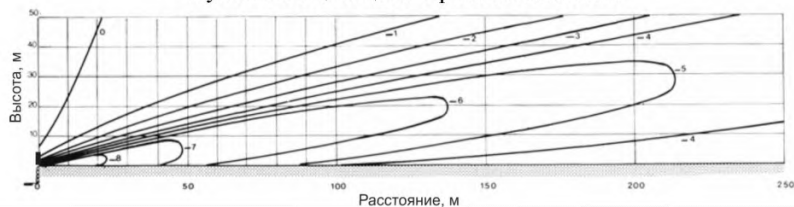
Рисунок В.6 - Распространение транспортного шума на территории, прилегающей к проектируемому участку четырехполосной дороги, расположенному в выемке с вертикальными откосами, в зависимости высоты экрана (цифры на кривых – снижение эквивалентных уровней транспортного шума, дБА)
