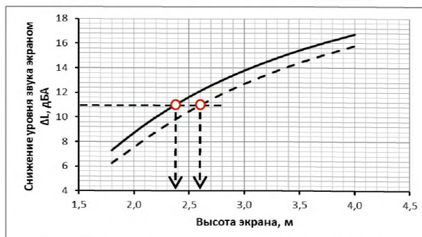
Рисунок Г.6 – Определение минимальной высоты экрана в расчетных сечениях
