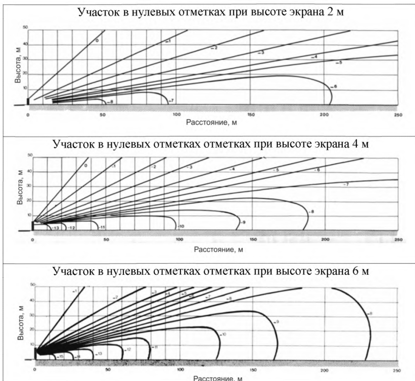
Рисунок В.3 - Распространение транспортного шума на территории , прилегающей к проектируемому участку четырехполосной дороги, в нулевых отметках в зависимости от высоты экрана (цифры на кривых – снижение эквивалентных уровней транспортного шума, дБА)
