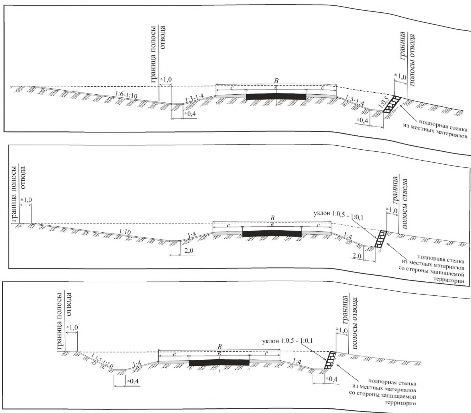
Рисунок 11.46 - Шумозащитные выемки
