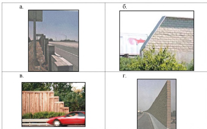
Рисунок 12.12 - Плавное, постепенное (а, б, в) и резкое изменение (г) высоты в начале (конце) экрана
