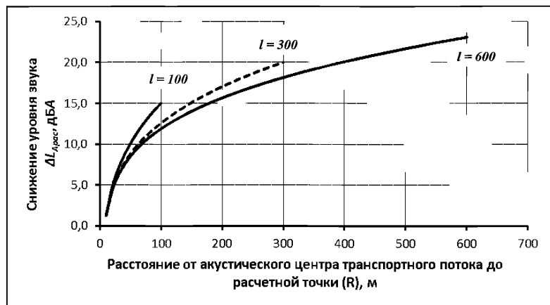
Рисунок Б.2 - Снижение уровня звука транспортного потока, в зависимости от увеличения расстояния до расчетной точки ( \Delta L_{Aрас} ) при длинах подлежащих расчету участков дороги ( l ) 100 м, 300 м и 600 м
