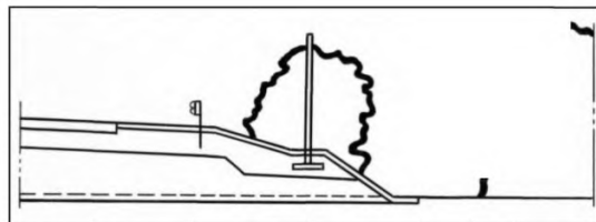
Рисунок 11.35 - Шумозащитный экран на дополнительной берме
