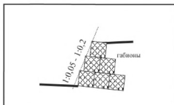
Рисунок 11.47 - Повышение устойчивости откосов шумозащитной выемки: армированный грунт, каменная кладка, габионы
