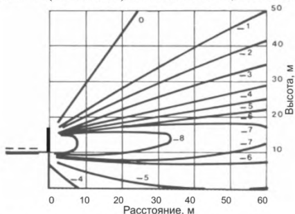
Рисунок В.7 - Распространение транспортного шума на территории, прилегающей к проектируемому участку шестиполосной дороги, в зависимости от высоты экрана и типа поперечного профиля (цифры на кривых – снижение эквивалентных уровней транспортного шума, дБА)
