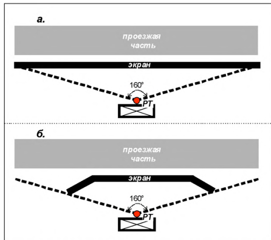
Рисунок 11.25 - Искривление экрана в сторону защищаемого участка (б) от источника шума позволяет уменьшить его общую длину 11.4.7.3 Схемы сокращения длины шумозащитного экрана
