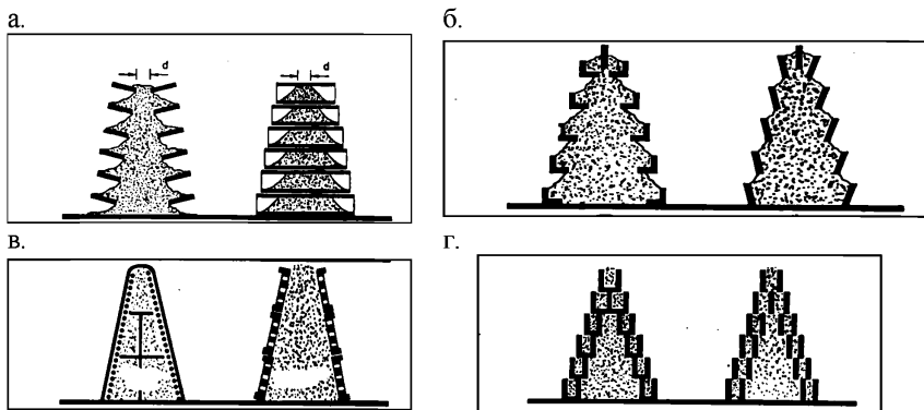
Рисунок 11.57- Конструкции комбинированных шумозащитных экранов: а – этажерка; б – применение уголковых элементов; в – решетчатая система; г – одевающие элементы
