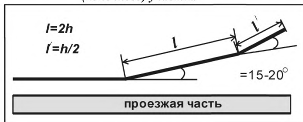
Рисунок 11.27 - Схема назначения параметров начального (конечного) участка
