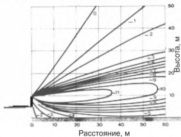
Рисунок В.2 - Снижение эквивалентных уровней транспортного шума на территории, прилегающей к проектируемому участку четырехполосной дороги, в зависимости от высоты экрана и поперечного профиля (цифры на кривых – снижение эквивалентных уровней транспортного шума, дБА)
