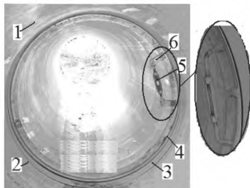
1 – труба; 2 – спигот; 3 – внутренняя поверхность спигота; 4 – обод струбцины; 5 – винтовая система; 6 – упор
