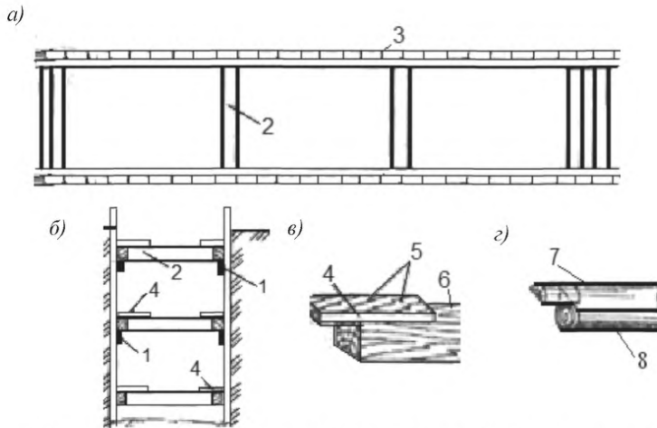
а) вид сверху; б) вид вдоль траншеи; в), г) узлы сопряжения элементов креплений
