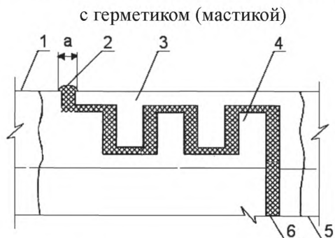
Рисунок 7.9 – Общий вид соединения ТПСС на винтовых выступах
