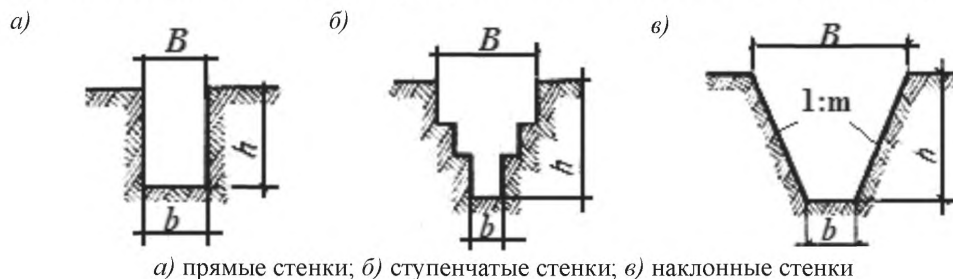
Рисунок 9.47 – Разрабатываемые многоковшовыми экскаваторами траншеи со стенками
