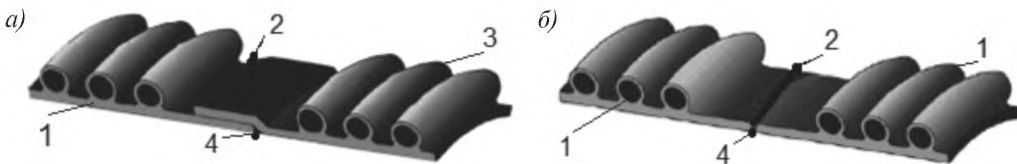
1 – трубы с гладким концом; 2, 4 – наружные и внутренние сварные швы; 3 – труба с раструбом Рисунок 7.12 – Фрагменты соединений спиральновитых из полых фигурного поперечного сечения профилей труб экструзионной сваркой гладкого конца в раструбе и гладких концов встык
