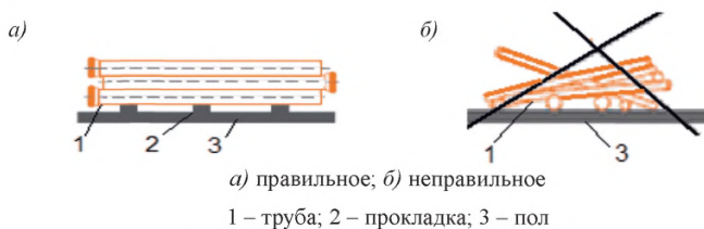
Рисунок 8.3 – Складирование ТПСС
