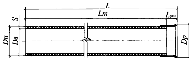
Рисунок 6.2 – Труба тип Б (из ТУ 2248-001-89628949-2010 [13])
