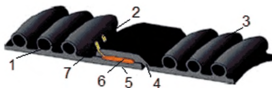
Рисунок 7.13 – Фрагмент раструба трубы из полиэтилена
