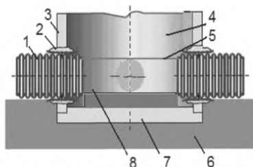
1 – труба; 2 – муфта с ЦПП; 3 – стенки; 4 – колодец; 5 – борма; 6 – грунт; 7 – днище колодца; 8 – лоток
