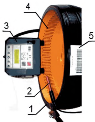
Рисунок 7.13 – Фрагмент раструба трубы из полиэтилена
