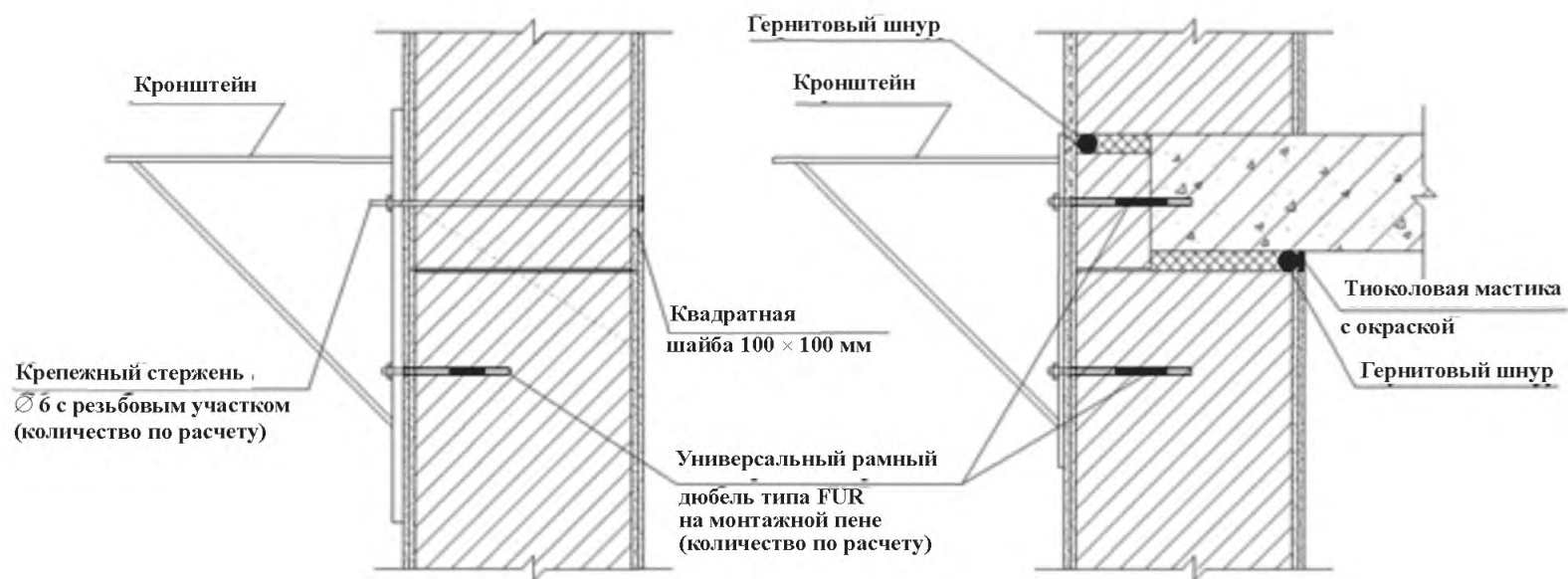
Устройство для крепления растяжек (при расчетном обосновании)
