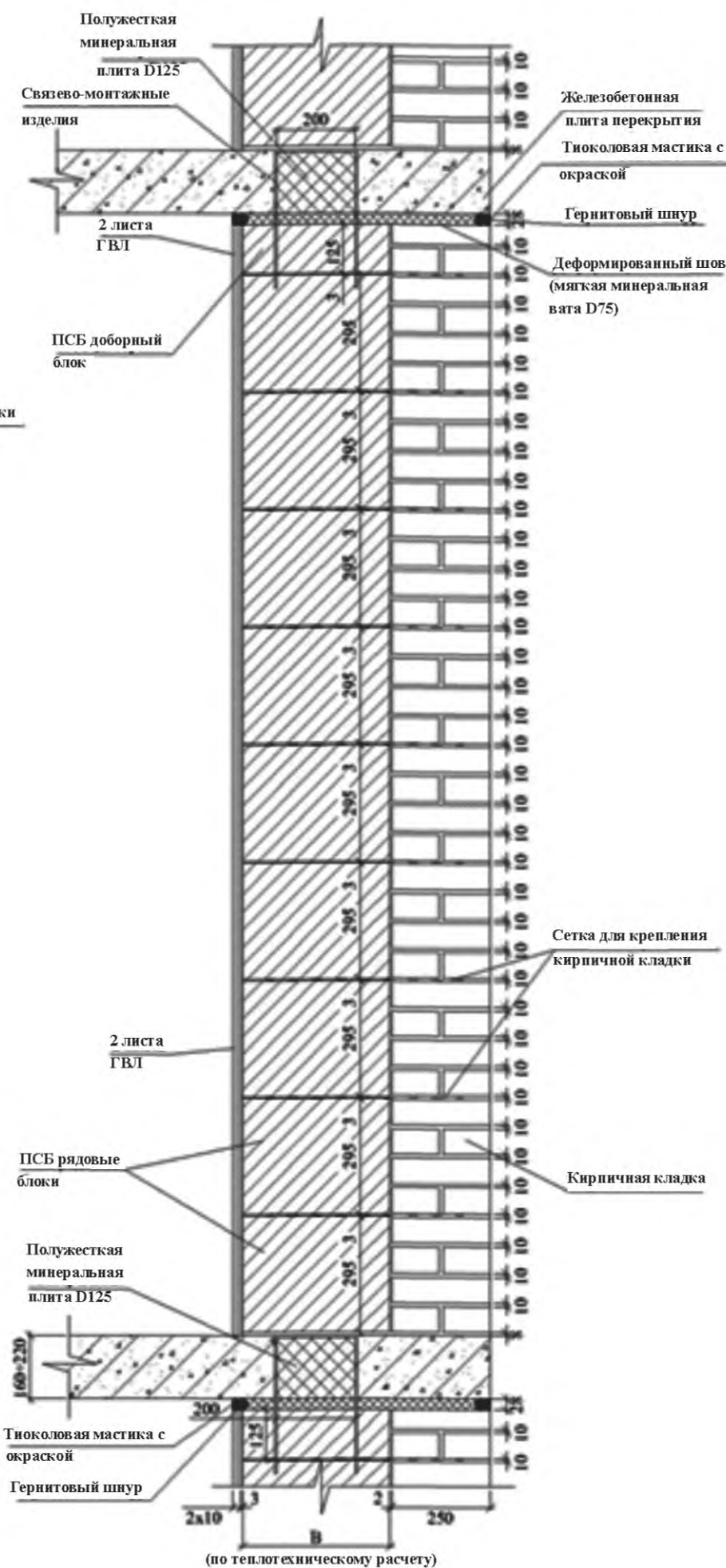
Рисунок 6.4 – Несущая стена из ПСУ блоков с наружной кирпичной облицовкой толщиной в 1 кирпич и внутренней облицовкой ГВЛ
