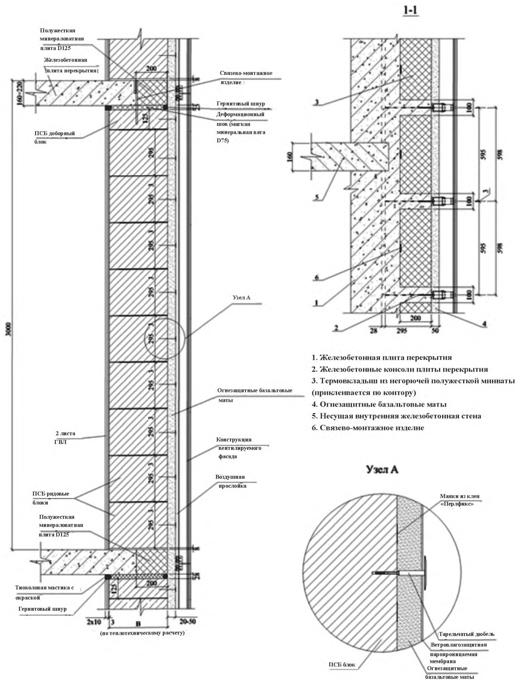
Рисунок 6.8, лист 2 – Ненесущая стена из ПСБ блоков с вентилируемым фасадом. Вертикальный разрез по глухому простенку и горизонтальный разрез по перекрытию
