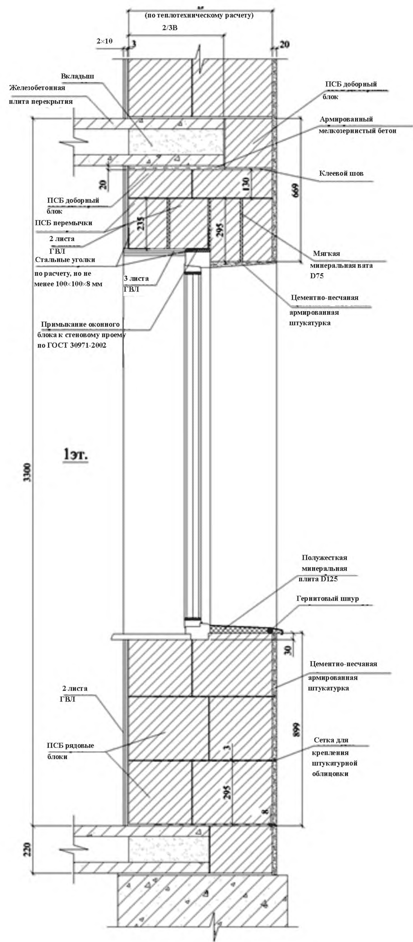
Рисунок 6.11 – Несущая стена из полистиролбетонных блоков с фасадной штукатуркой. Вертикальный разрез по оконному проему
