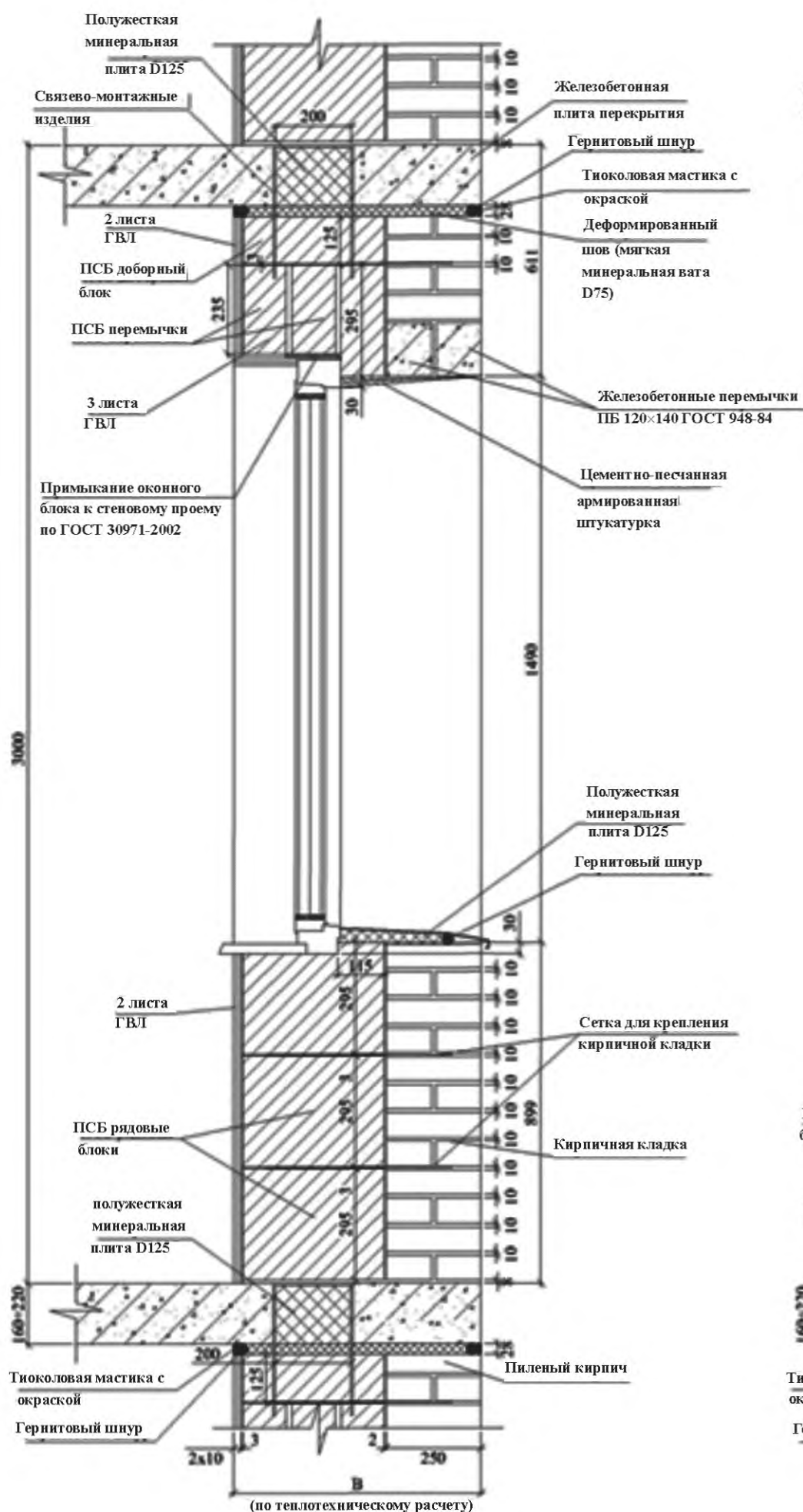
Рисунок 6.4 – Несущая стена из ПСУ блоков с наружной кирпичной облицовкой толщиной в 1 кирпич и внутренней облицовкой ГВЛ
