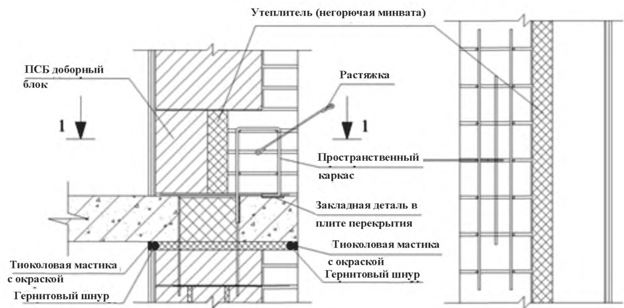
Устройство для крепления растяжек к кирпичному фасаду
