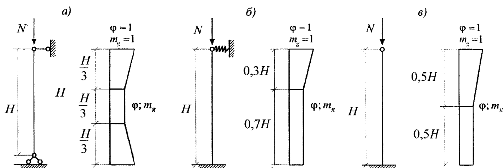
а) – шарнирно опертые на неподвижные опоры внизу и вверх; б) – защемленные внизу и с упругой опорой вверх; в) – защемленные внизу и свободные вверх
