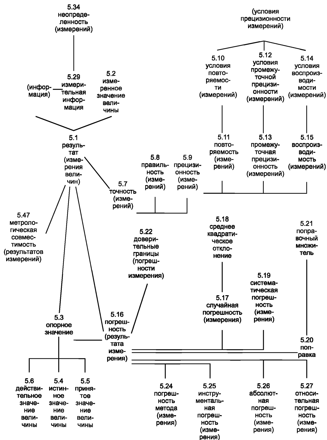
Рисунок 4 – Схема к разделу 5 для терминов, связанных с понятием «точность измерений»
