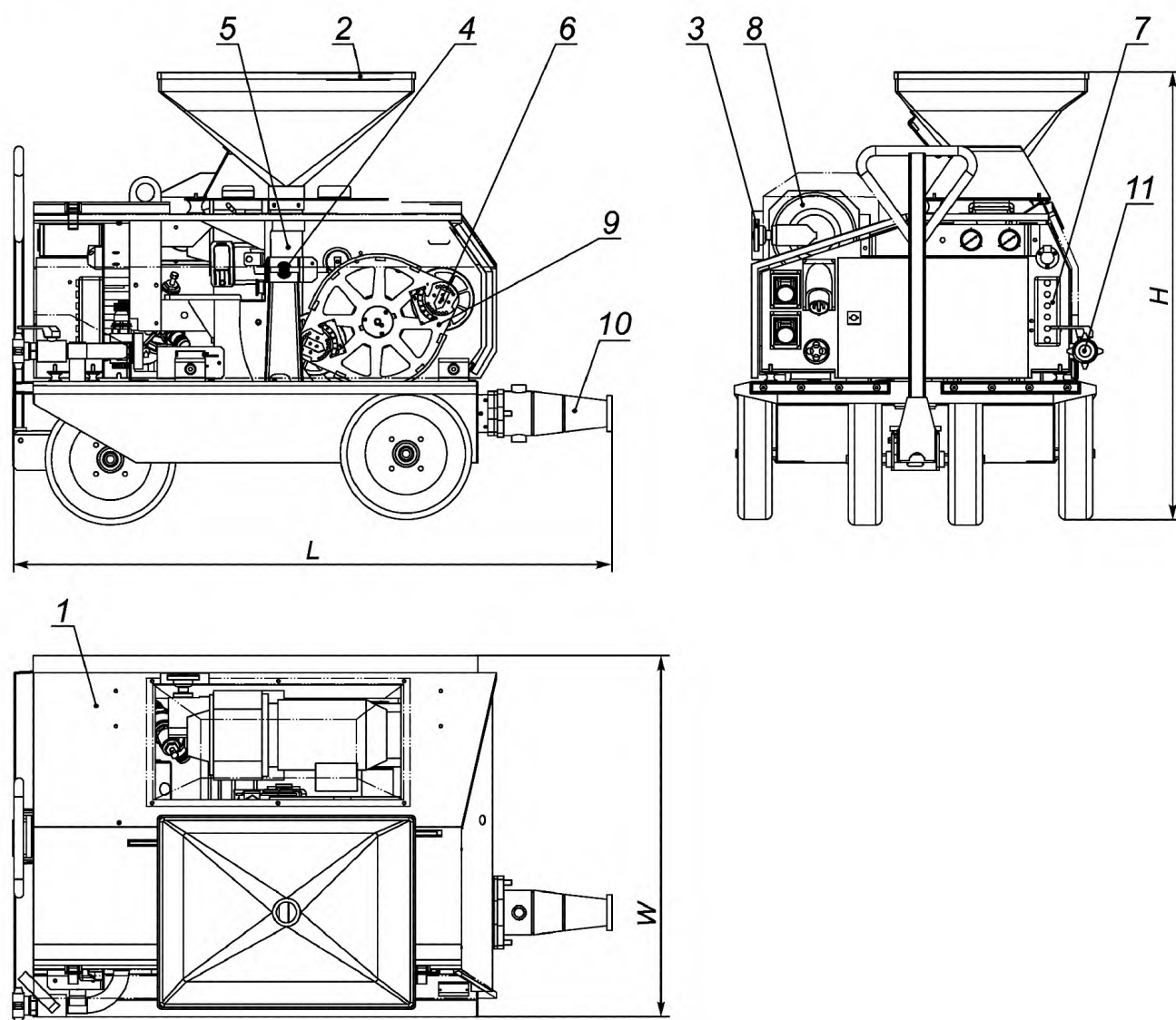
а) Габаритные размеры.
