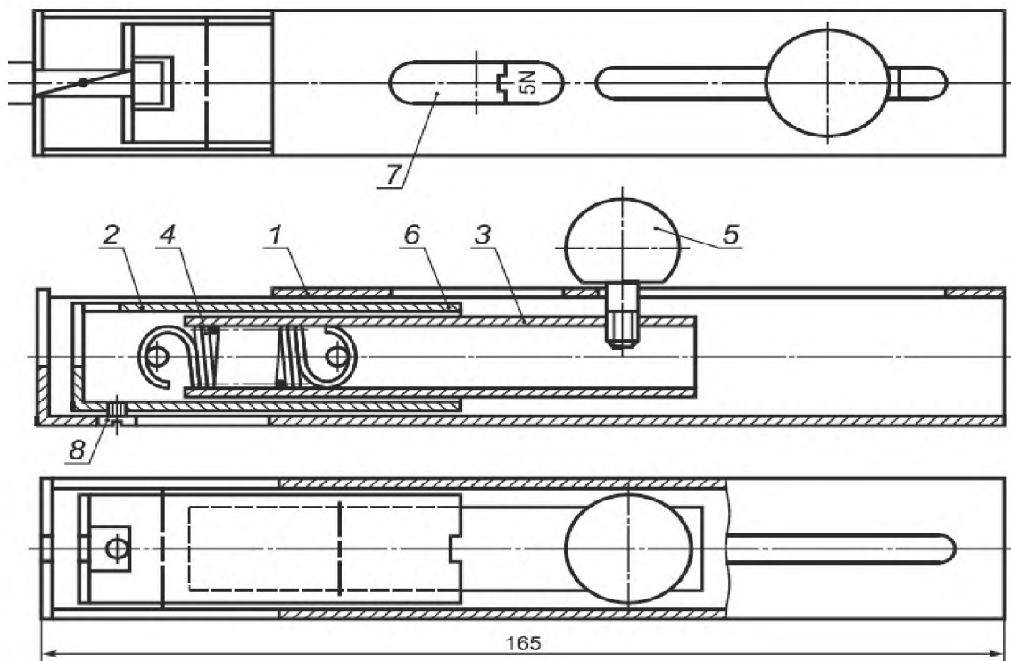
Рисунок 7 — Испытательное приспособление для приложения в осевом направлении растягивающей силы
