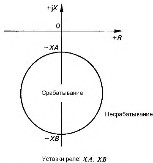
Рисунок 1ф — Круговая смещенная характеристика
