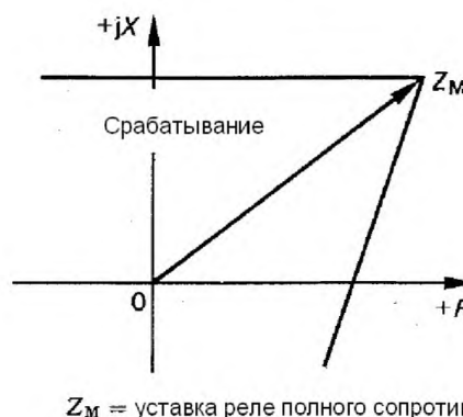
Рисунок 1б — Характеристика реактивного сопротивления
