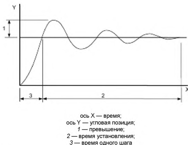
Рисунок 1 — Наибольшее значение и время установления
