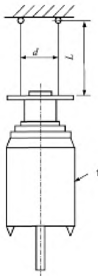
1 — ротор
