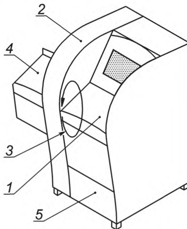
1 — подающее устройство с загрузочным лотком; 2 — кожух ножа; 3 — вращающийся серповидный или дисковый нож; 4 — разгрузочный лоток; 5 — поддон для сбора крошек
