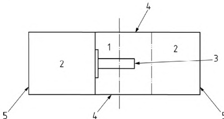
1 — зона 1; 2 — зона 2; 3 — режущее устройство в переднем положении; 4 — несъемное защитное ограждение ( h_{\min} = 300 мм); 5 — рама машины ( h_{\min} согласно EN ISO 13857)
