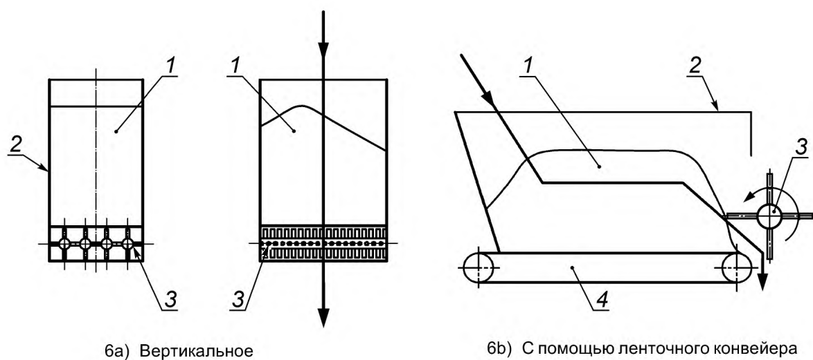
1 — тесто; 2 — емкость для теста; 3 — разгрузитель; 4 — ленточный конвейер
