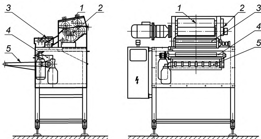
Рисунок 28 — Опасные зоны машины для нарезания заготовок из теста
