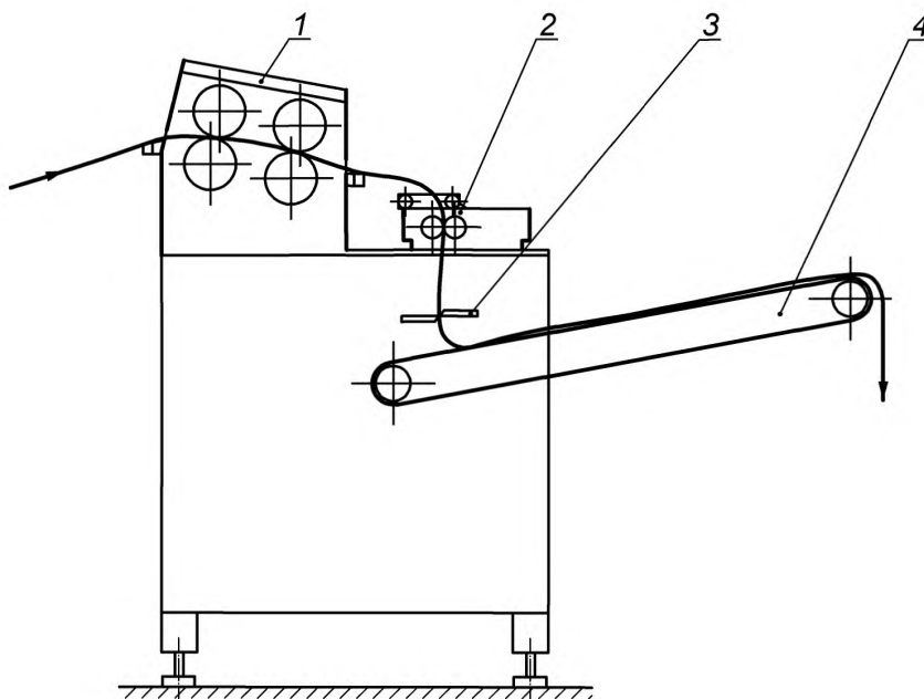
1 — валец для калибровки толщины заготовок из теста; 2 — блок продольного нарезания; 3 — нож для поперечной резки; 4 — конвейер
