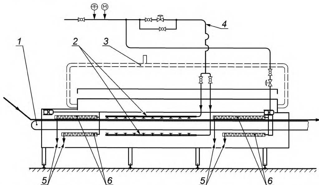
1 — конвейер; 2 — трубы обработки паром; 3 — система удаления пара; 4 — система подвода пара; 5 — сбор конденсата; 6 — отопительные рукава
