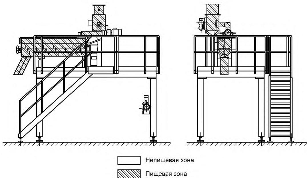
Рисунок 32 — Тестомесильная машина непрерывного действия
