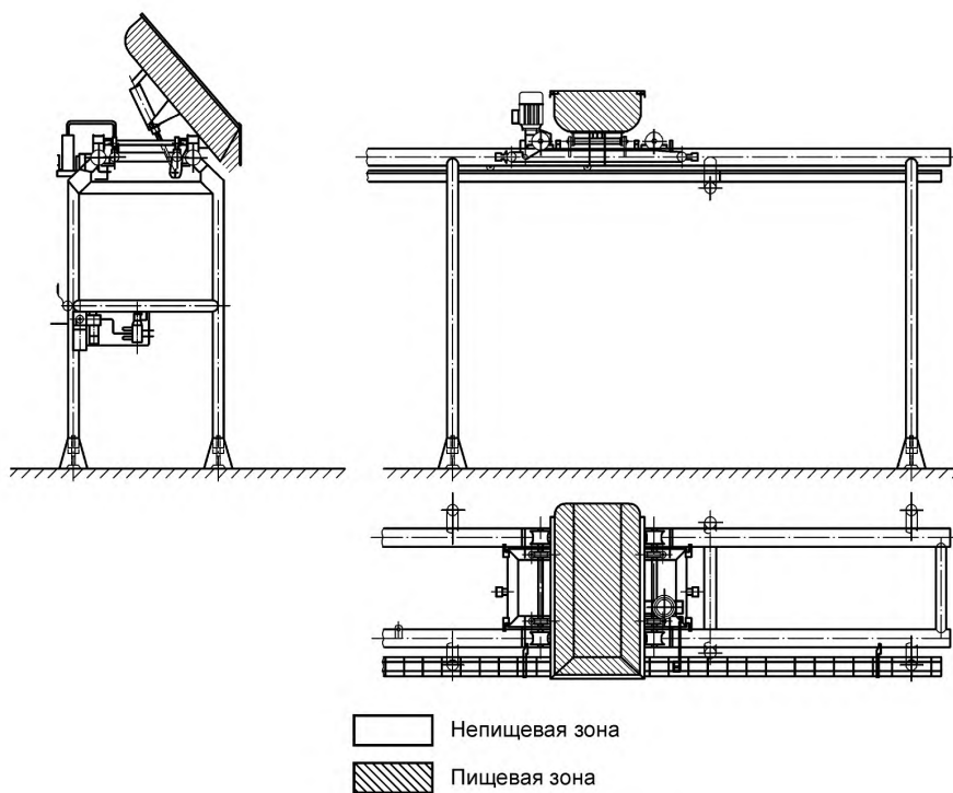
Рисунок 38 — Транспортёр емкости для теста
