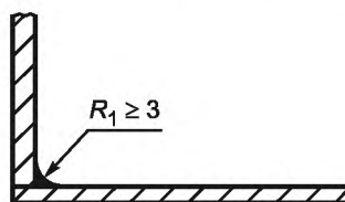
Рисунок В.2 — Пищевая зона
