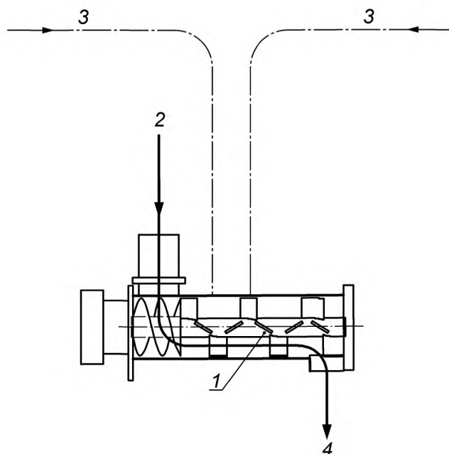
1 — вал с лопастями; 2 — отверстие для загрузки измельченных продуктов; 3 — отверстие для загрузки жидкостей; 4 — отверстие для выгрузки продуктов
