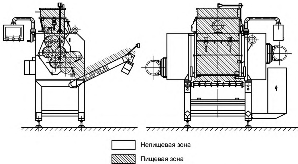
Рисунок 36 — Формовочная машина заготовок из теста
