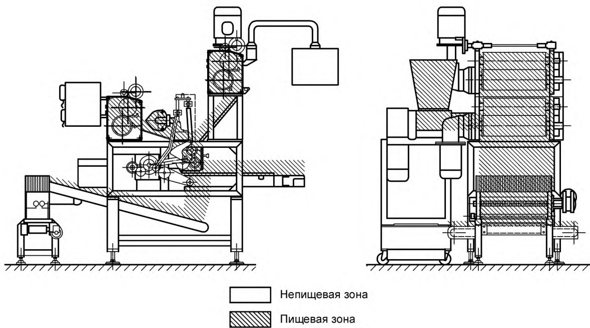
Рисунок 35 — Формовочная машина изделий из теста для обработки двух заготовок из теста
