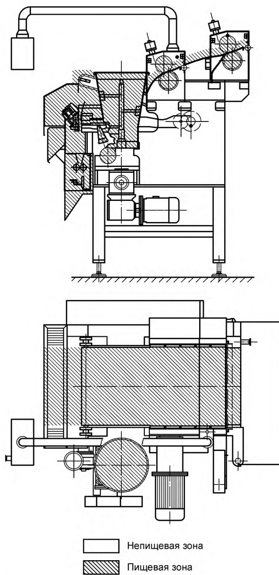
Рисунок 34 — Формовочная машина изделий из теста
