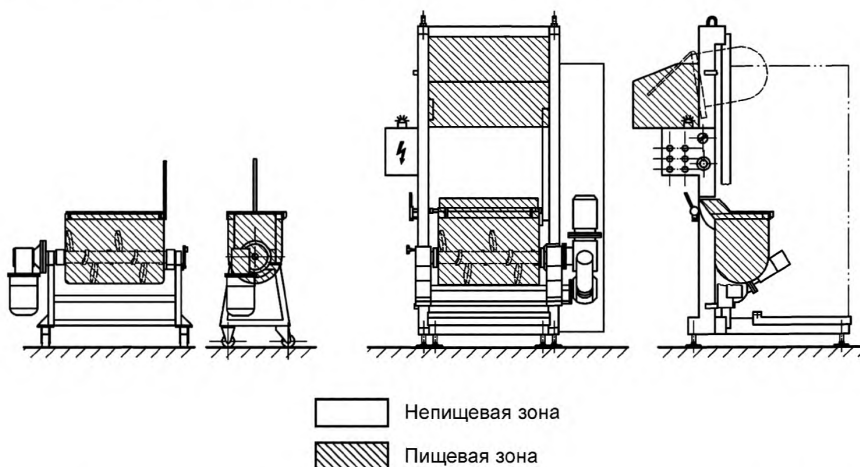
Рисунок 31 — Тестомесильная машина периодического действия, загружаемая вручную, с подъемным устройством или без него и опрокидывающим устройством или без него
