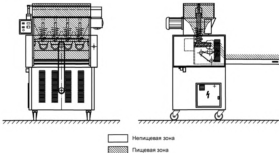
Рисунок 43 — Машина для производства макаронных изделий
