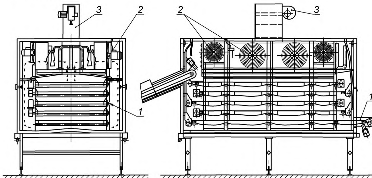
Рисунок 27 — Опасные зоны охладителя
