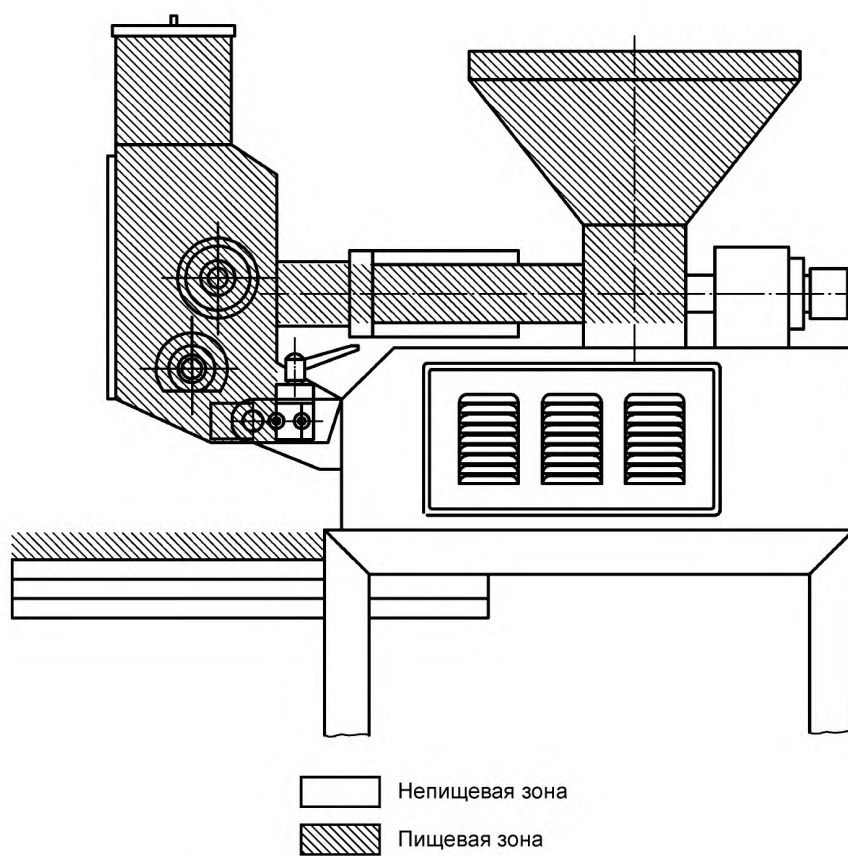
Рисунок 42 — Машина для производства ньокки
