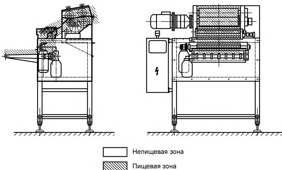
Рисунок 41 — Машина для нарезки заготовок из теста
