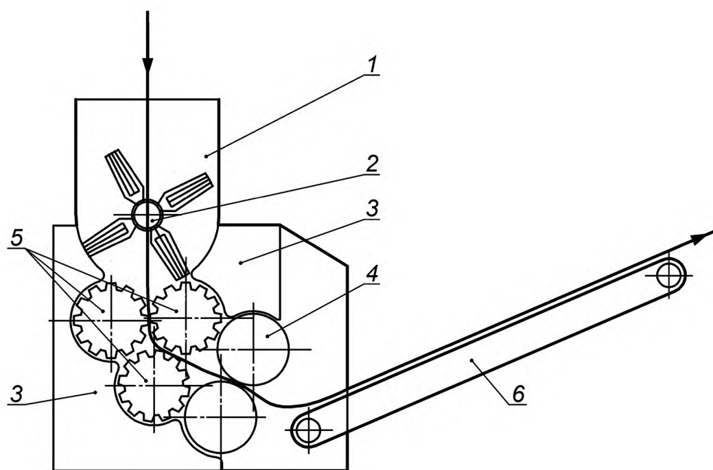
1 — бункер; 2 — вал с лопастями; 3 — изогнутые емкости; 4 — вальцы для тонкой калибровки; 5 — вальцы для нарезания; 6 — ленточный конвейер
