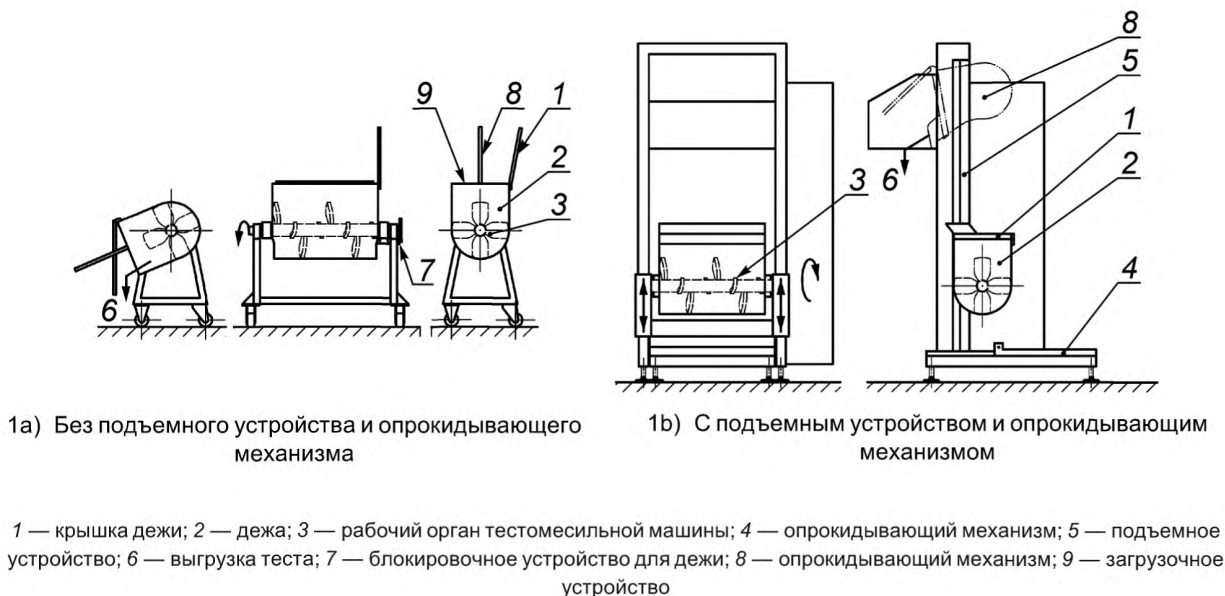
Рисунок 1 — Тестомесильная машина периодического действия, загружаемая вручную
