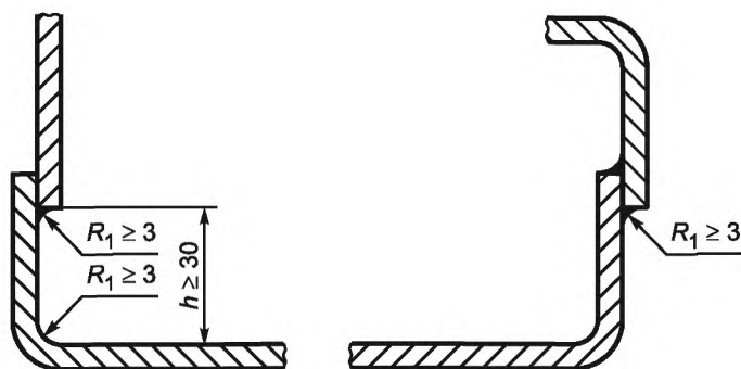
Рисунок В.7 — Пищевая зона
