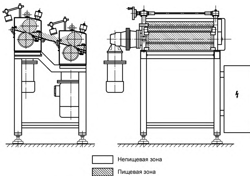
Рисунок 37 — Вальцовая машина для калибровки заготовок из теста
