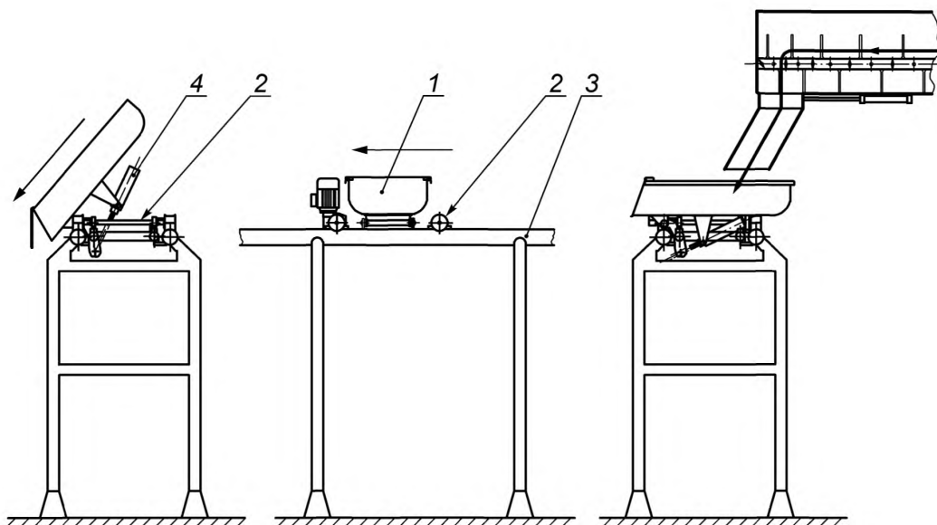
1 — лоток; 2 — транспортер; 3 — рама с направляющими; 4 — устройство опрокидывания
