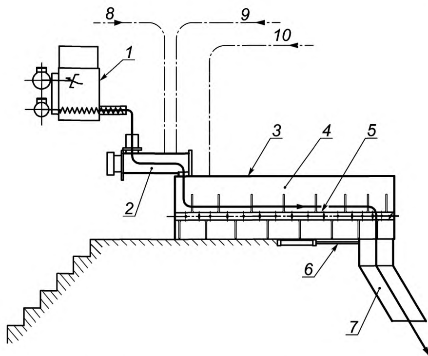
1 — дозатор для муки, крупы и других измельченных продуктов; 2 — устройство предварительного замешивания; 3 — крышка дежи; 4 — дежа; 5 — вал с лопастями; 6 — отверстие для выгрузки теста; 7 — воронка; 8 — отверстие для подачи яиц; 9 — отверстие для подачи жидкости; 10 — отверстие для подачи остатков теста
