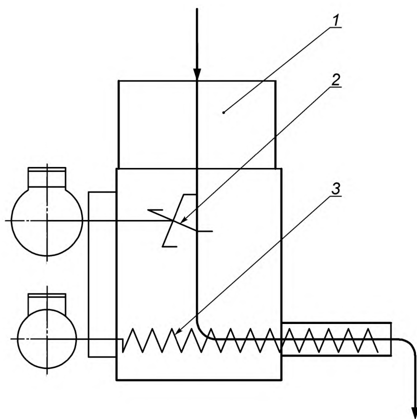
1 — воронка; 2 — вибратор; 3 — дозировочный шнек
