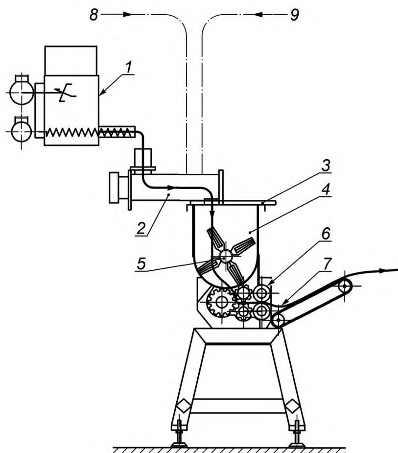
1 — дозатор для муки; 2 — смеситель для предварительного замешивания; 3 — крышка дежи; 4 — дежа; 5 — месильный орган с лопастями; 6 — валец; 7 — ленточный конвейер; 8 — отверстие для подачи яиц; 9 — дозатор жидкостей
