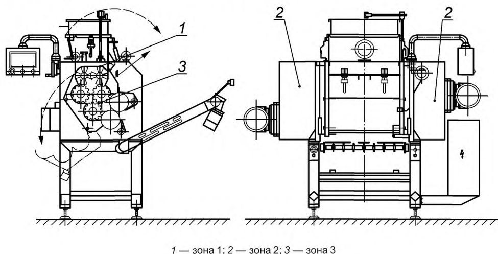
Рисунок 23 — Опасные зоны формовочной машины заготовок из теста
