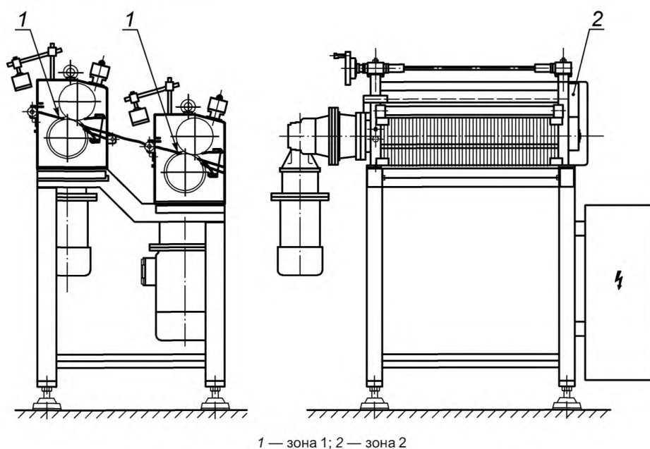
Рисунок 24 — Опасные зоны калибровочной машины
