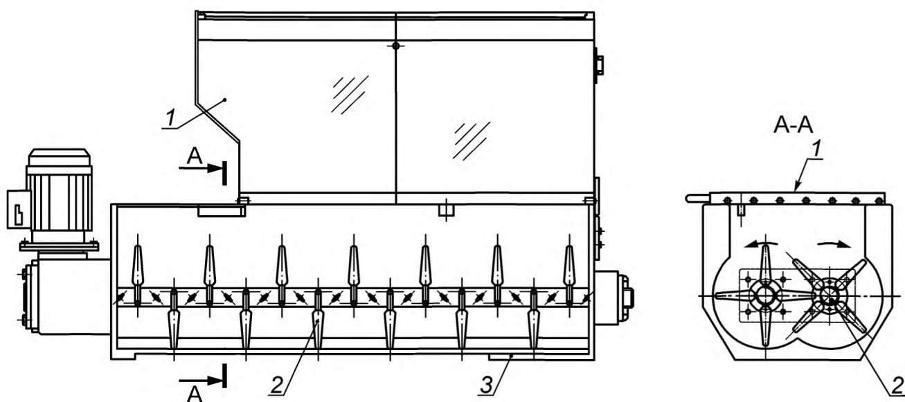
3а) С валом для замешивания
