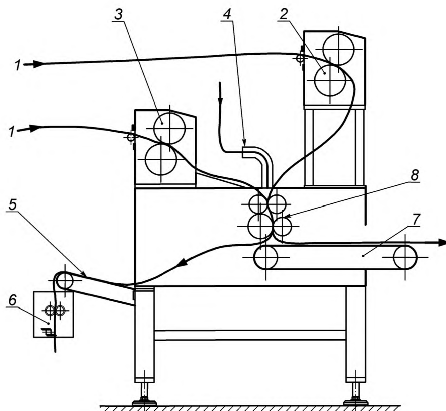
1 — подача заготовок из теста; 2 — калибровочные вальцы для верхних заготовок из теста; 3 — калибровочные вальцы для нижних заготовок из теста; 4 — устройство заполнения; 5 — устройство для сбора остатков теста; 6 — резак остатков теста; 7 — желоб сбора продуктов; 8 — формовочный узел
