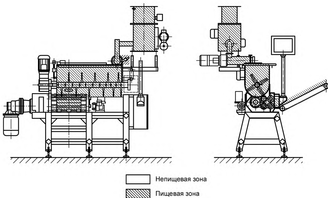
Рисунок 33 — Комбинирование тестомесильной машины и формовочной машины для заготовок из теста
