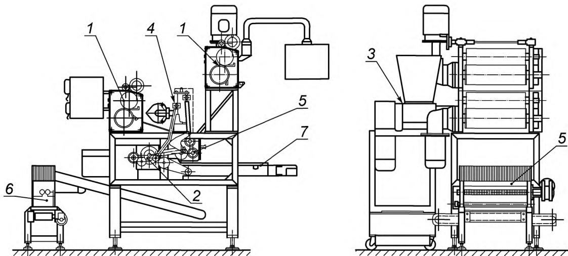
Рисунок 22 — Опасные зоны формовочной машины для обработки двух полосок из теста
