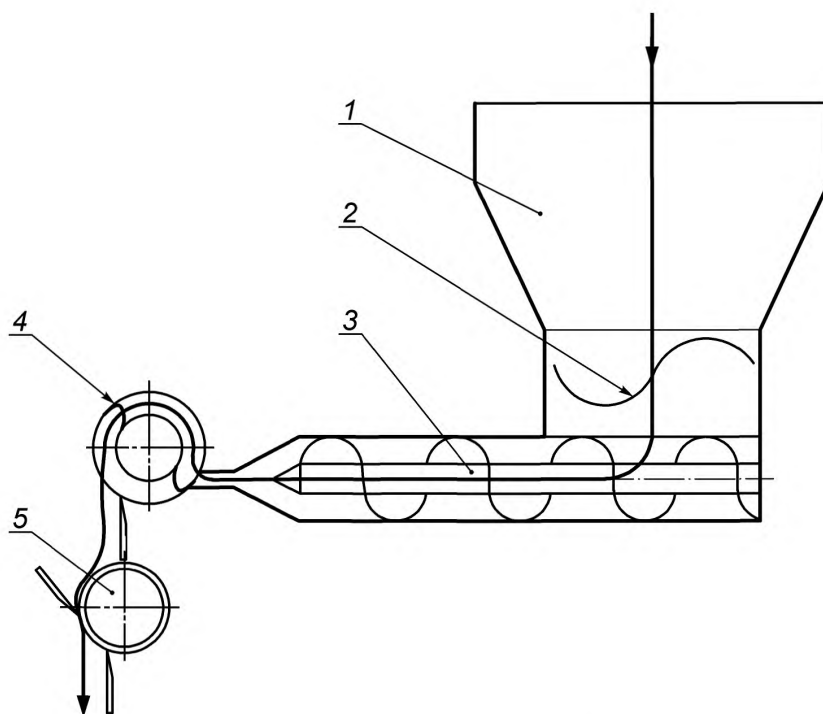
1 — бункер; 2 — рыхлитель; 3 — шнек; 4 — вращающиеся ножи; 5 — формовочные вальцы
