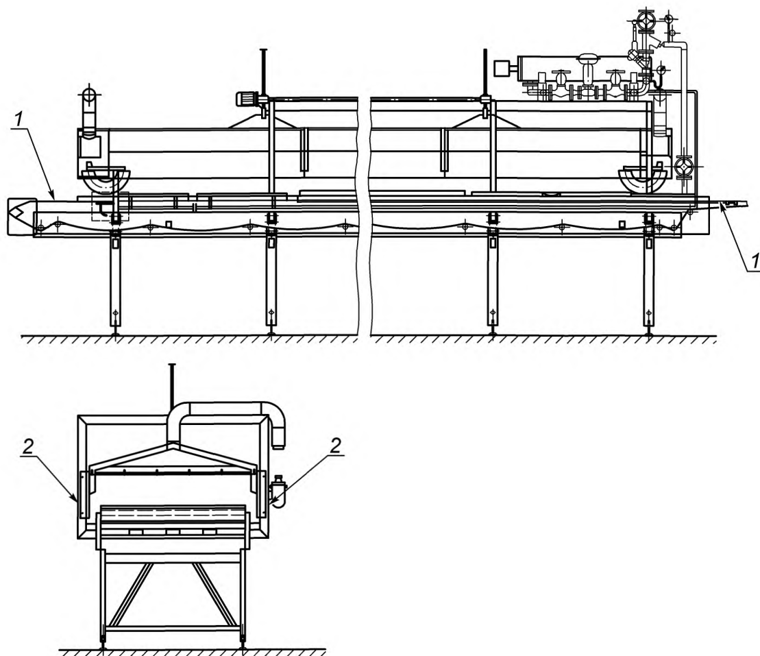
Рисунок 26 — Опасные зоны пастеризатора
