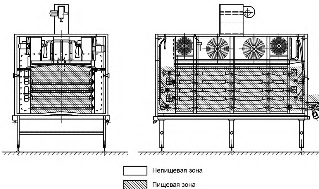
Рисунок 40 — Охладитель
