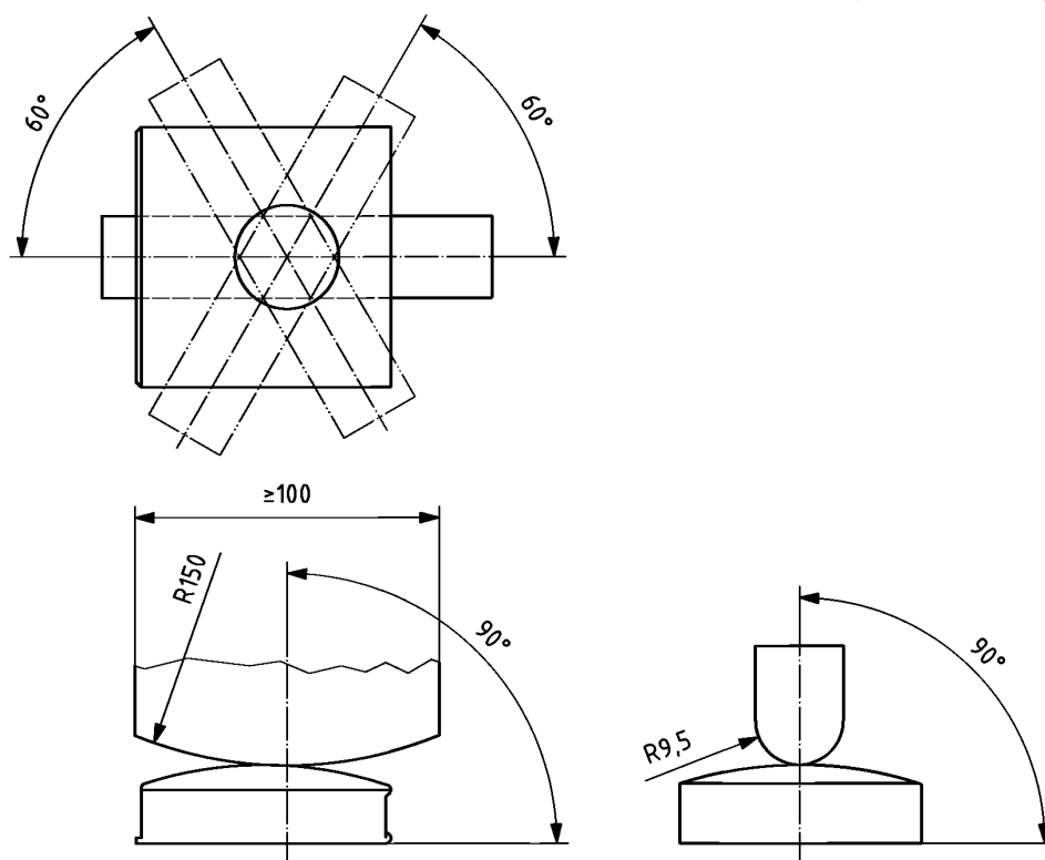
Рисунок 4 — Сжатие пряжки
