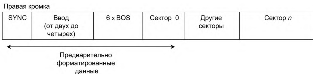
Рисунок 6 — Структура дорожки с неполной записью, секторы типов 0—5
