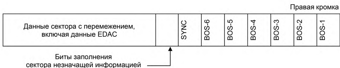
Рисунок 8 — Структура сектора, типы 0—5
