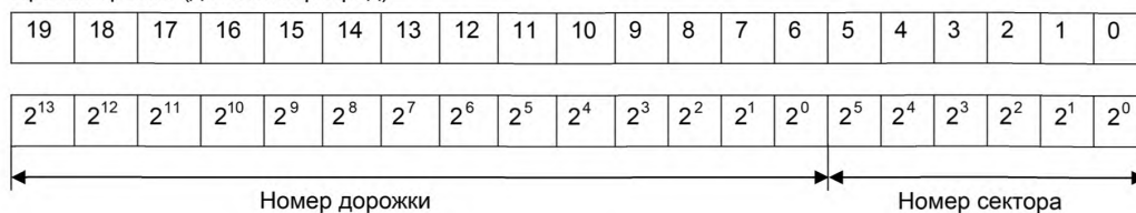
Рисунок 4 — Формат адреса сектора и дорожки
