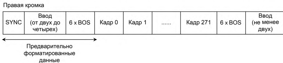
Рисунок 7 — Структура дорожки (с полной и частичной записью) для секторов с максимальным перемежением, типы 7—15
