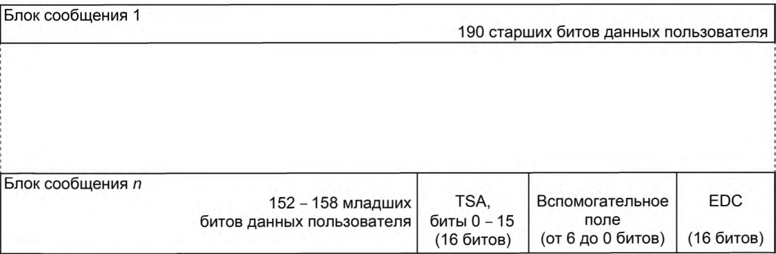
Рисунок 12 — Данные сектора до применения кода EDAC (для секторов всех типов, за исключением типа 5)
