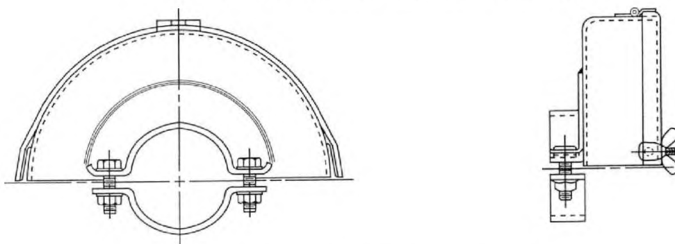
Рисунок 102a – Пример а) защитного кожуха
