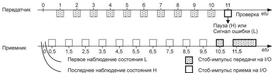
Рисунок 10 — Временные соотношения сигнала ошибки
