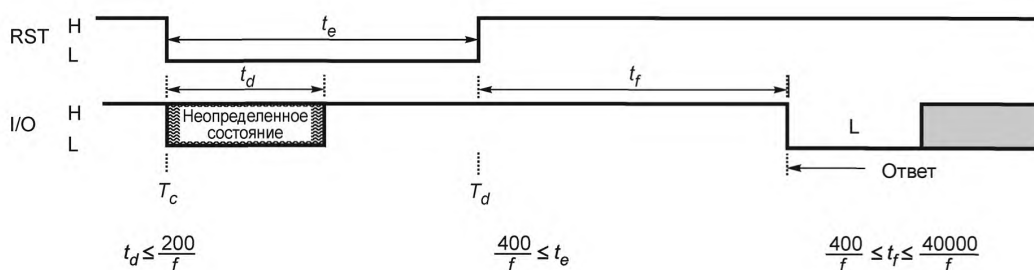
Рисунок 2 — «Горячее» восстановление
