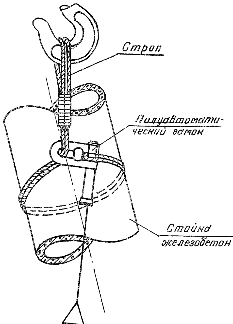
Рис. 6. Схема строповки железобетонной стойки полуавтоматическим стропом с захватом Смеля (Узел А).
