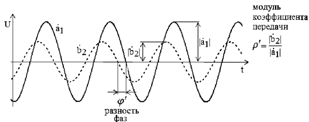
Рисунок A.12 – Представление напряжений прошедшей и падающей волн при измерении комплексного коэффициента передачи во временной области
