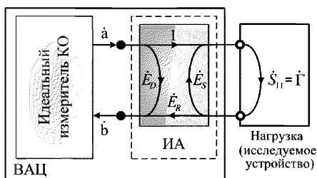
Рисунок А.4 – Модель ВАЦ (рефлектометра)
