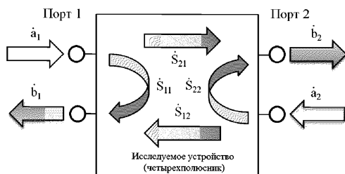
Рисунок А.8 – Распространение сигналов при измерении двухпортового устройства (четырепольника)
